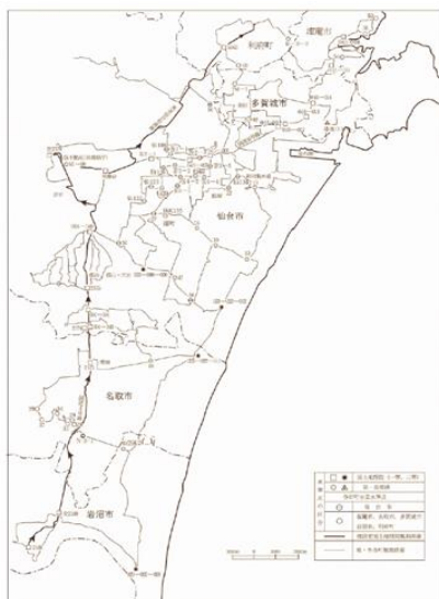
▲ 図3-4-3-1 仙台平野地域水準測量観測路線
