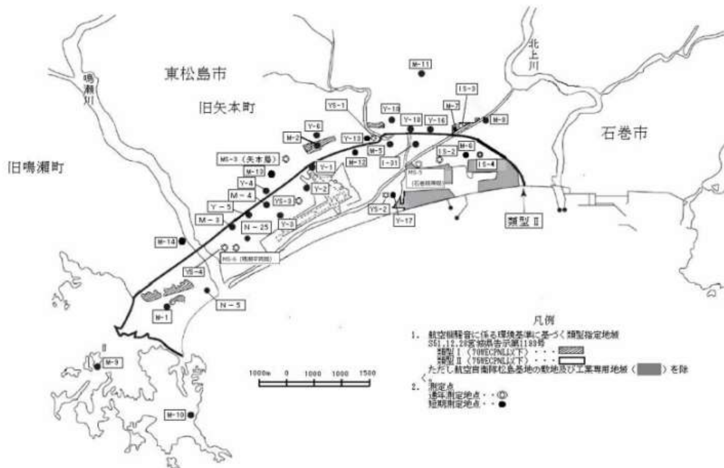
図3-4-4-2 航空自衛隊松島飛行場周辺航空機騒音測定地点
