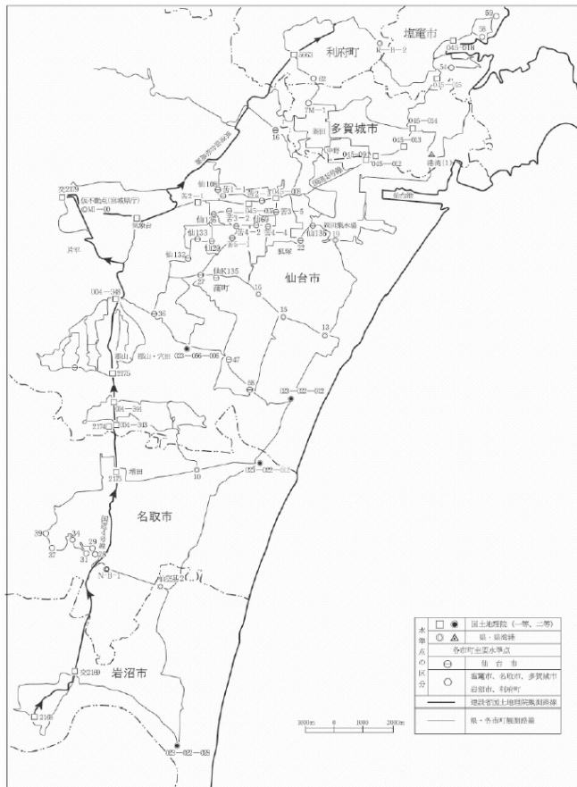
図2-4-3-1 仙台平野地域水準測量観測路線
