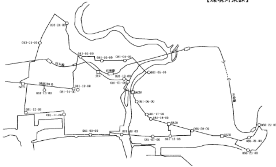
図2-4-3-4 石巻地域水準測量観測路線
