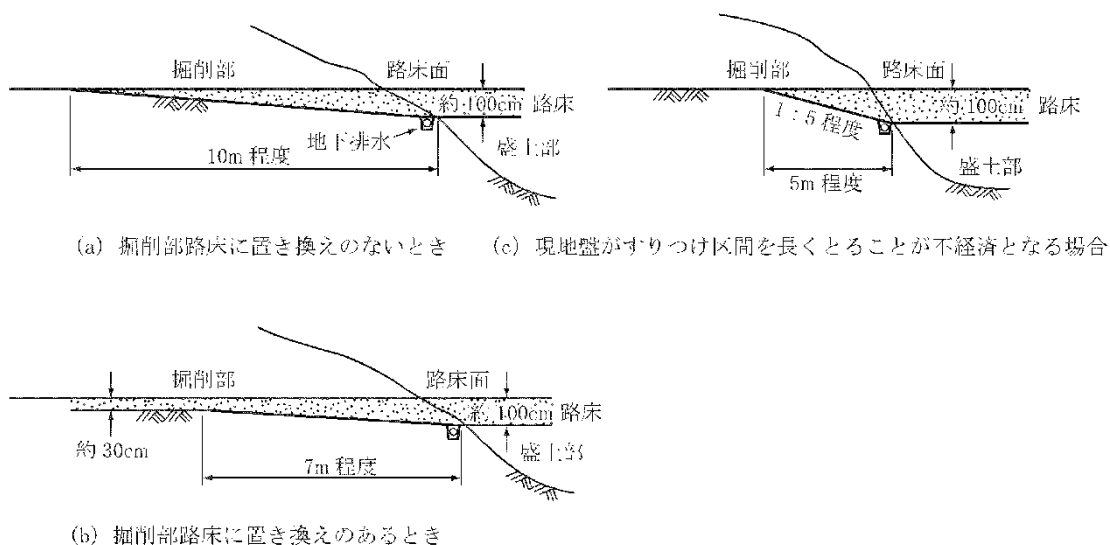
図2-3 掘削（切土）部、盛土部接統部のすり付け
