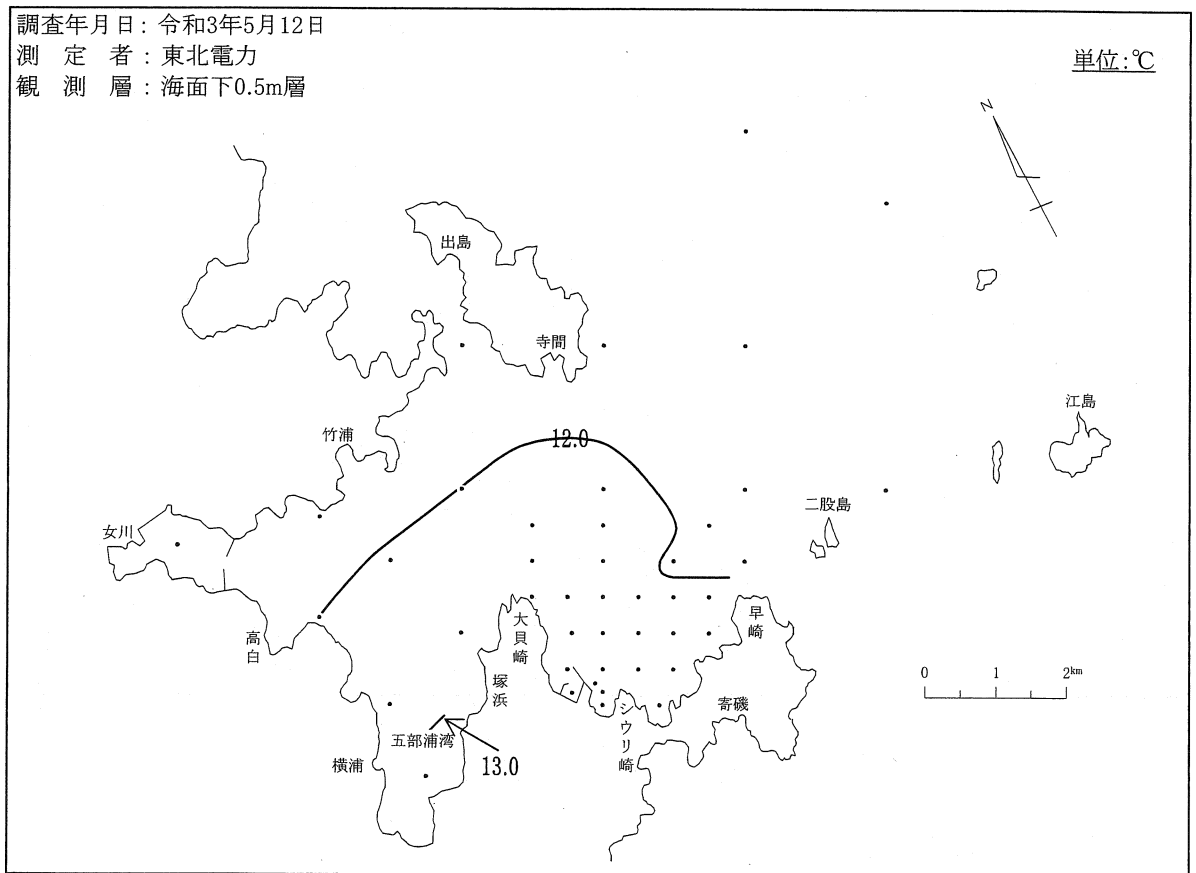
図-4-(2) 等温線
