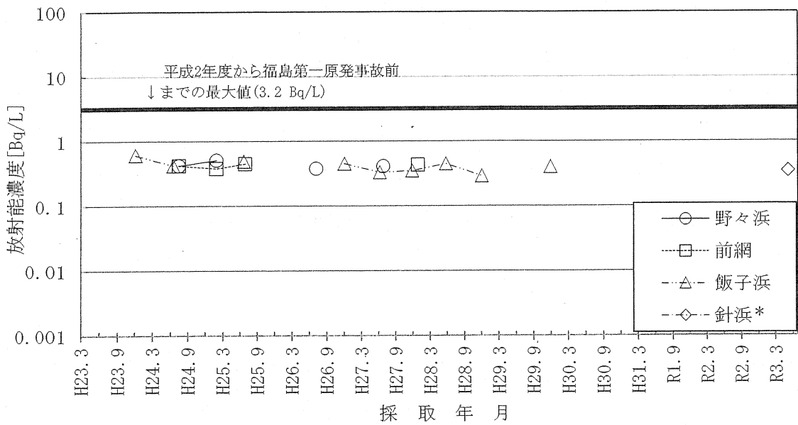
図-2-30 陸水のH-3濃度の推移
