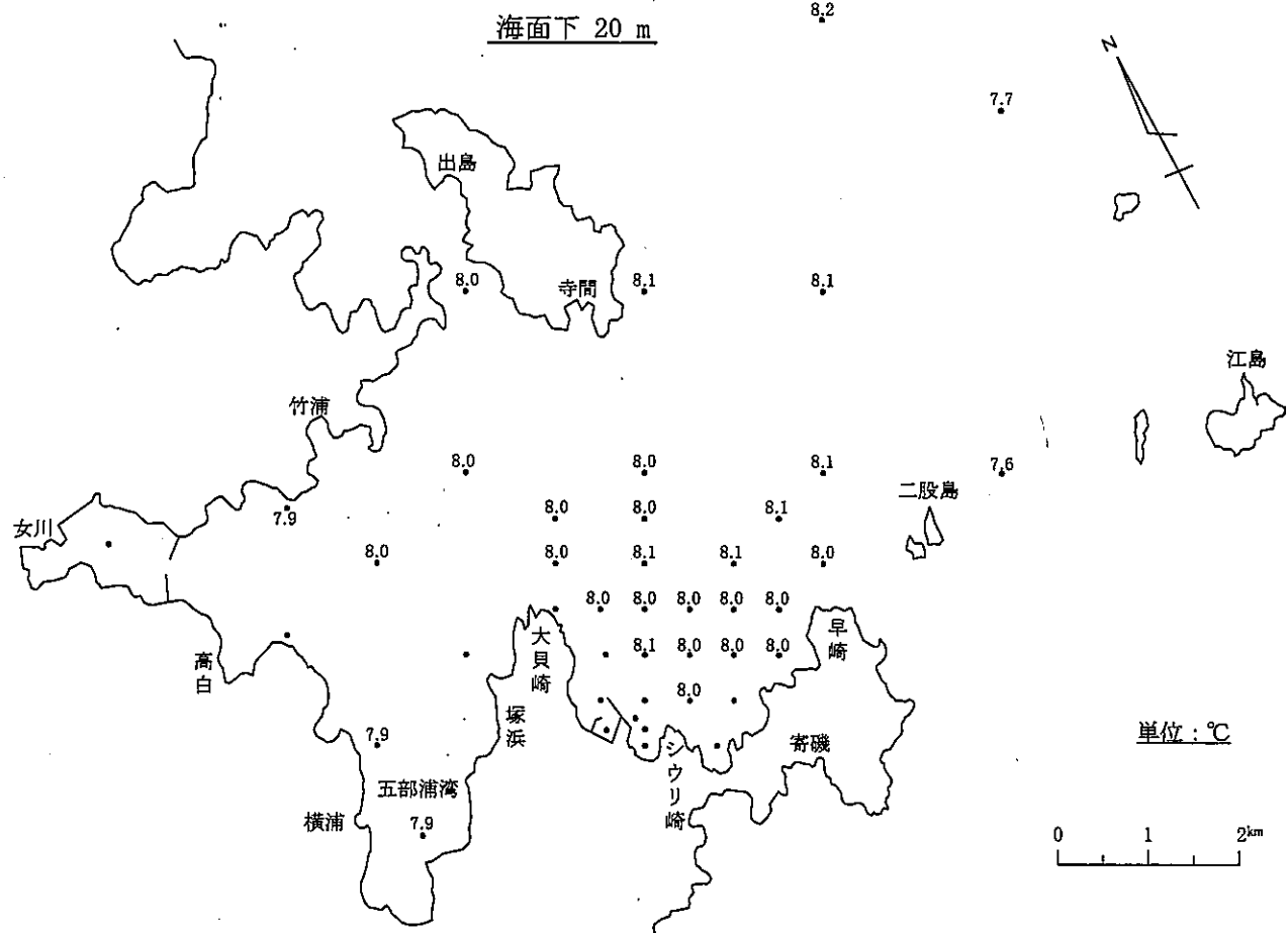
図-12-(2) 水温水平分布
