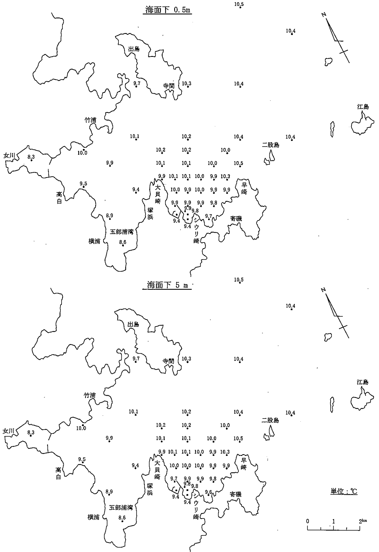
図-11-(1) 水温水平分布
