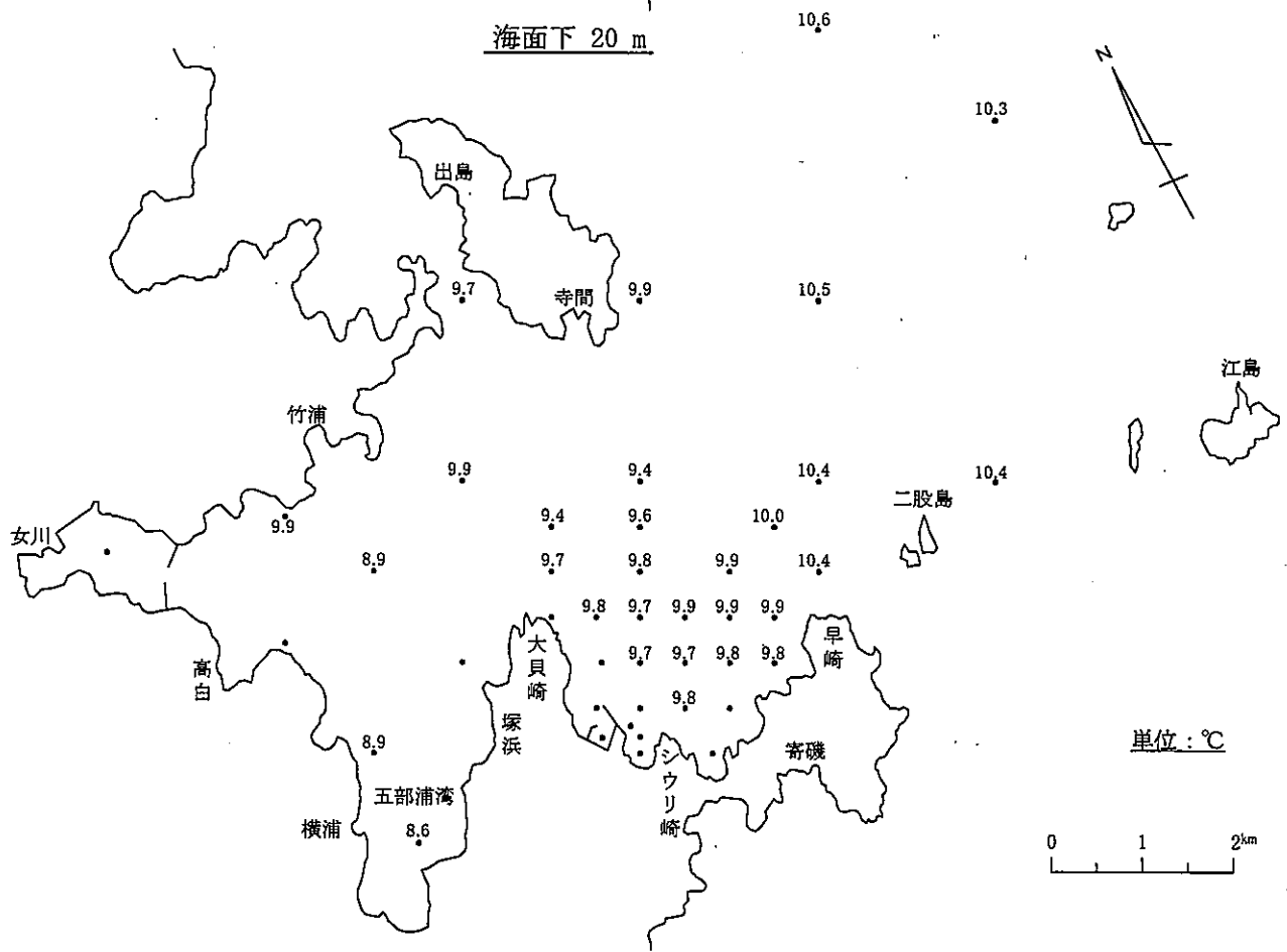
図-11-(2) 水温水平分布
