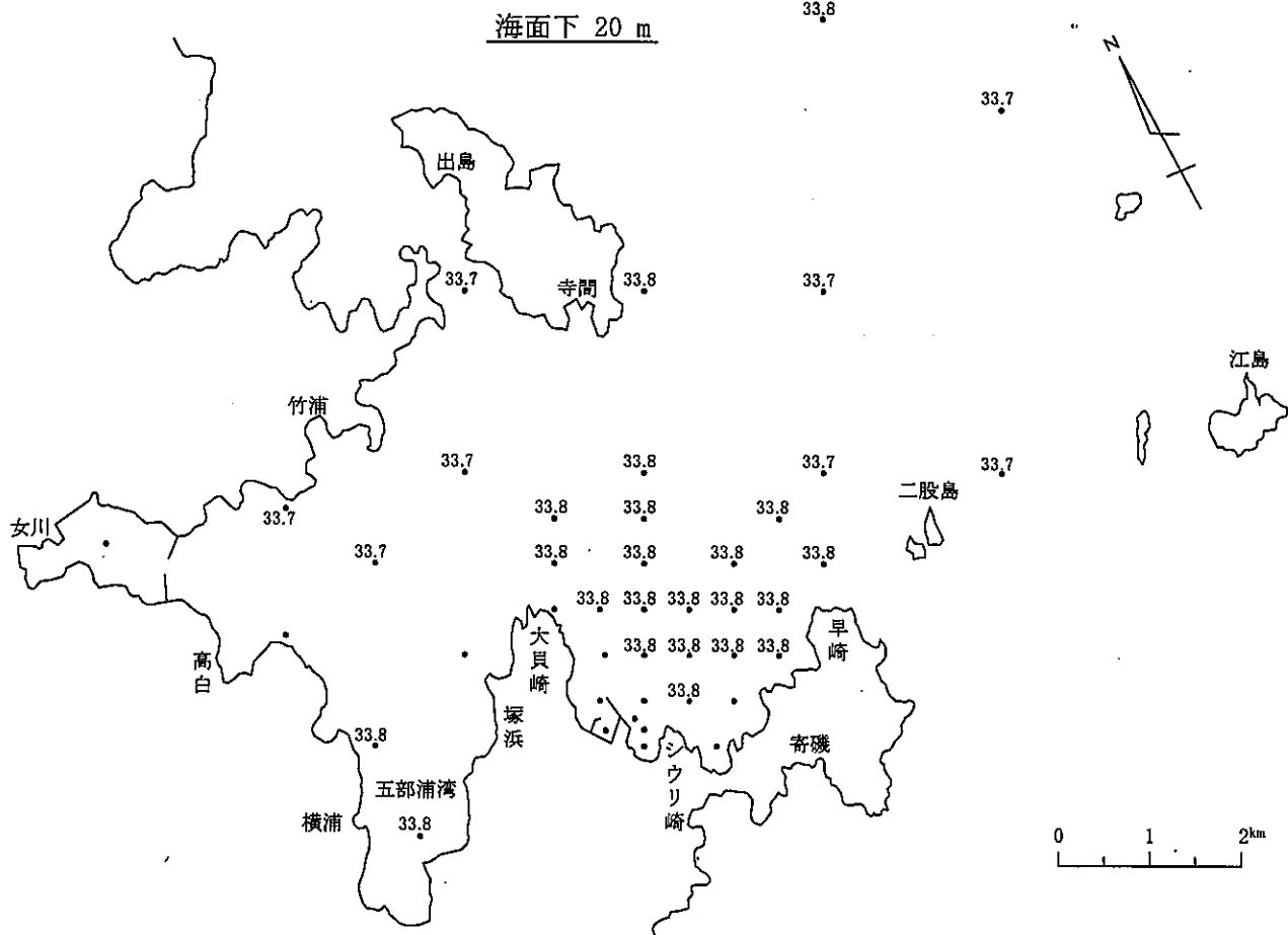
図-14-(2) 塩分水平分布
