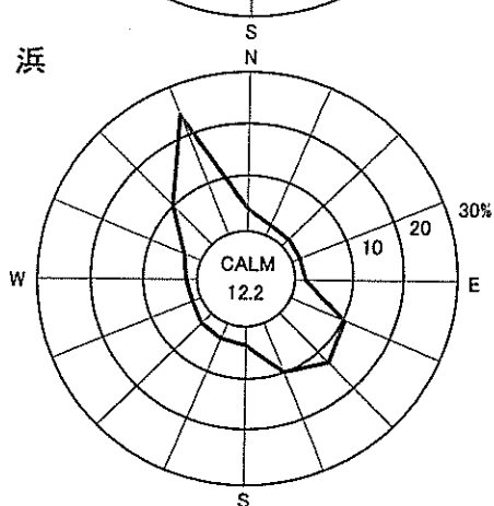
図-4-1-1 年間風配図(宮城県調査分)
