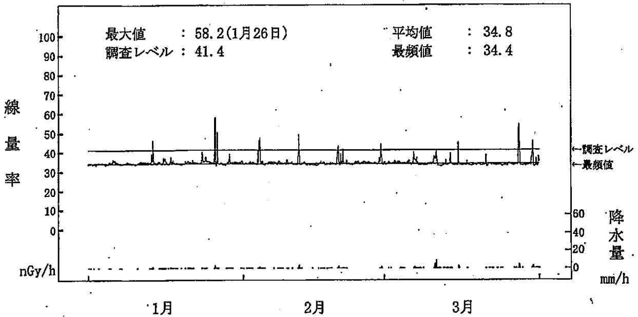
図-2-6 空間ガンマ線線量率監視結果 (江島局) (注) 3月6日の欠測は、定期点検によるものである。
