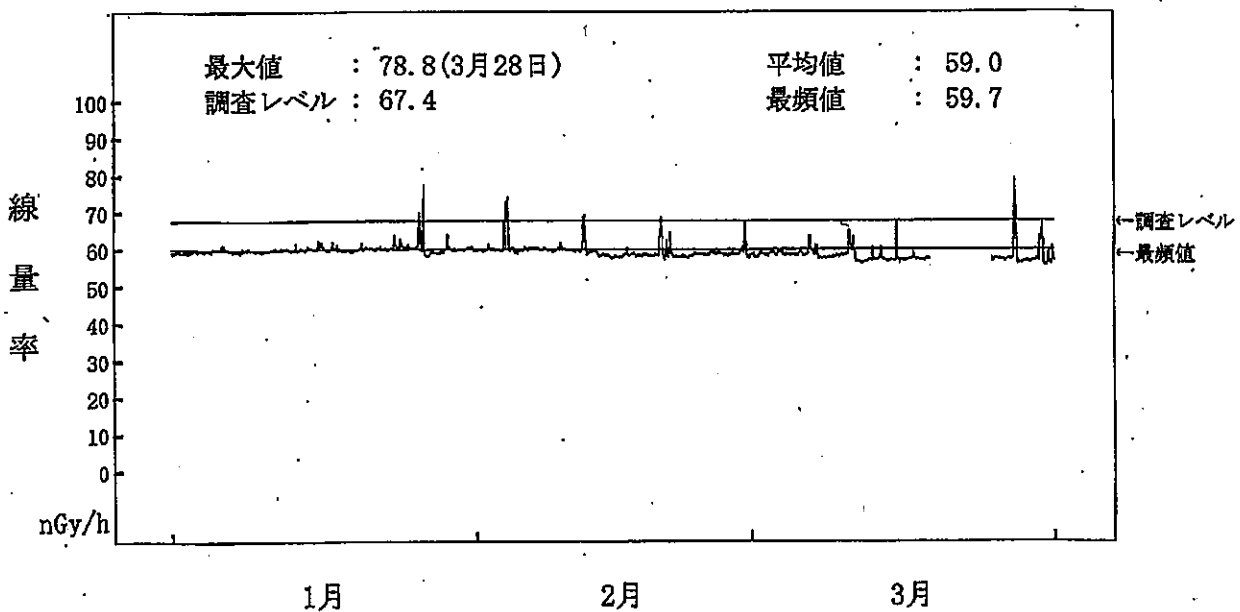
図-2-7 空間ガンマ線線量率監視結果 (前網局) (注) 3月19日~25日の欠測は、非常用発電機設置工事によるものである。
