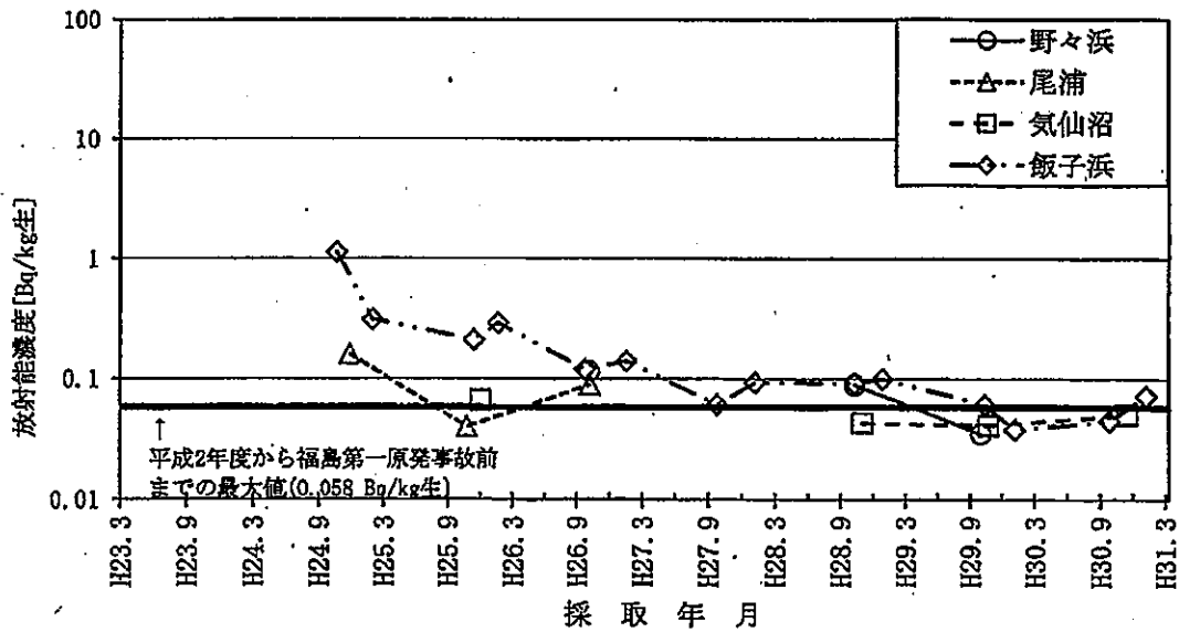
図-2-17 カキのCs-137濃度の推移
