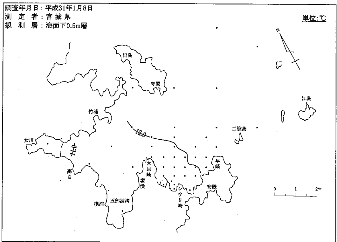
図-2-(2) 等温線
