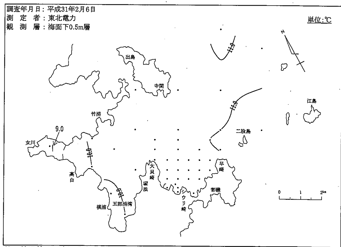
図-4-(2) 等温線
