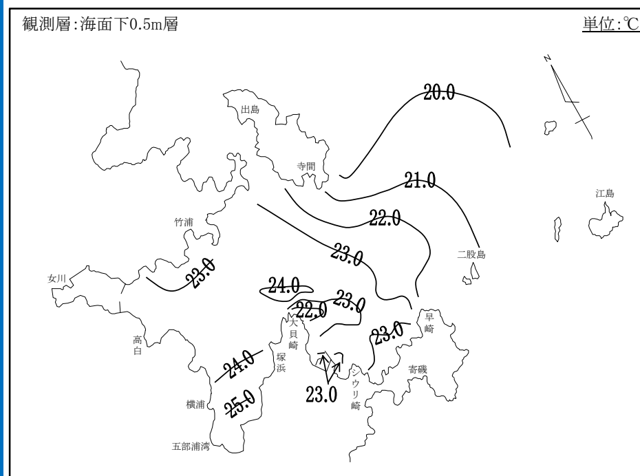
今回水温水平分布図 (平成29年7月11日)
