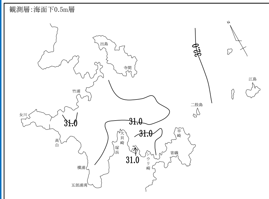
今回塩分水平分布図 (平成29年7月11日)
