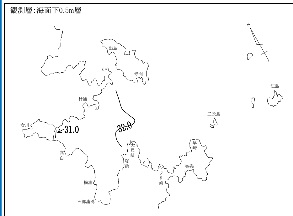
今回塩分水平分布図 (平成29年8月7日)
