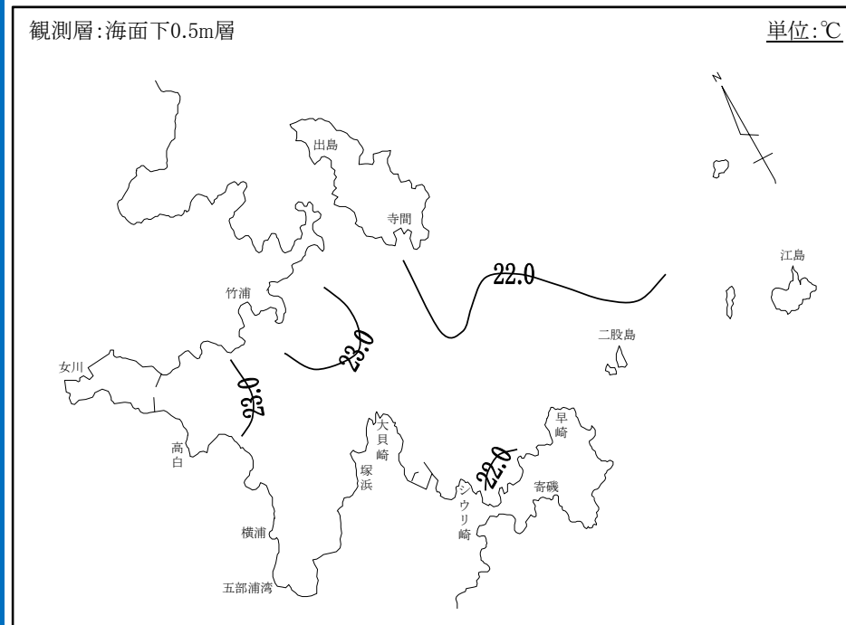
今回水温水平分布図 (平成29年8月7日)
