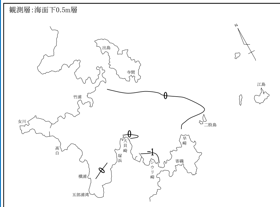
等値線 (今回塩分と平年塩分との差)
