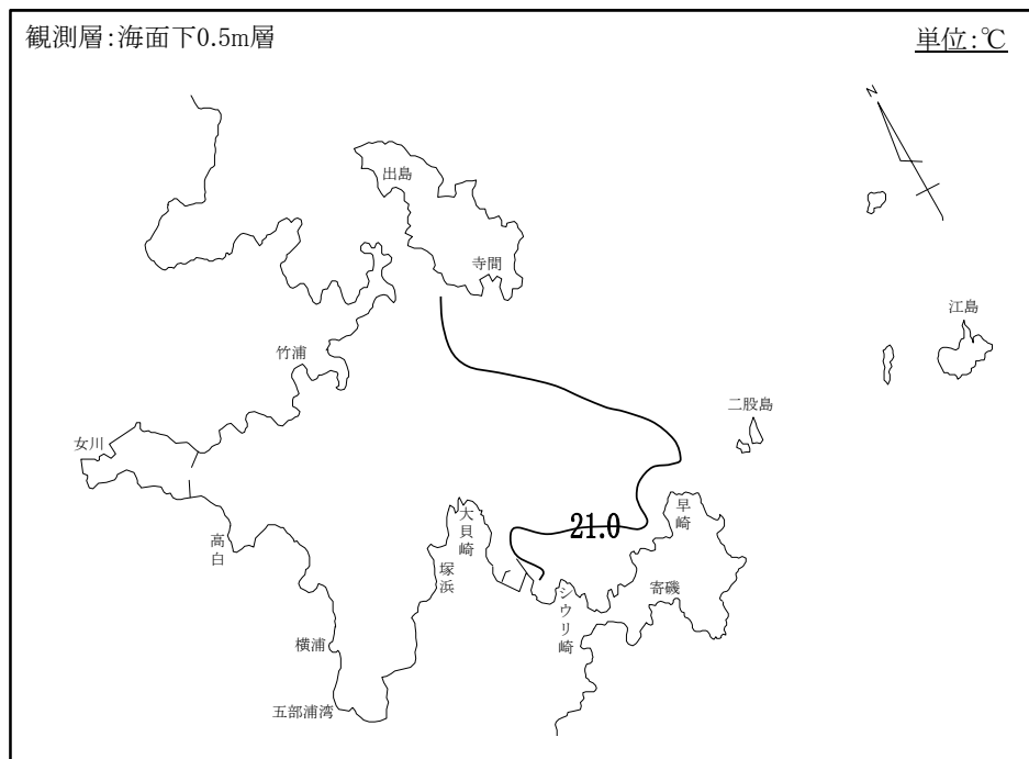
平年水温水平分布図 (昭和60年～平成28年)
