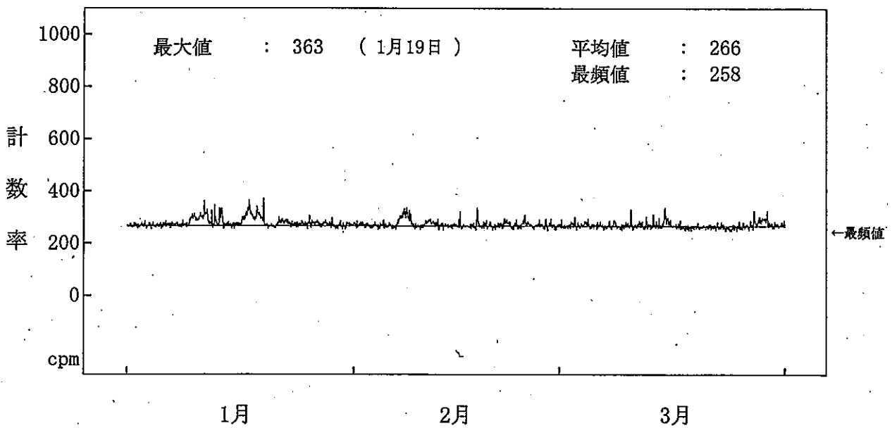
図一 2 - 9 海水(放水)中の全ガンマ線計数率監視結果(1号機放水口モニター(B)) (注) 2月16日の欠測は、停電作業によるものである。
