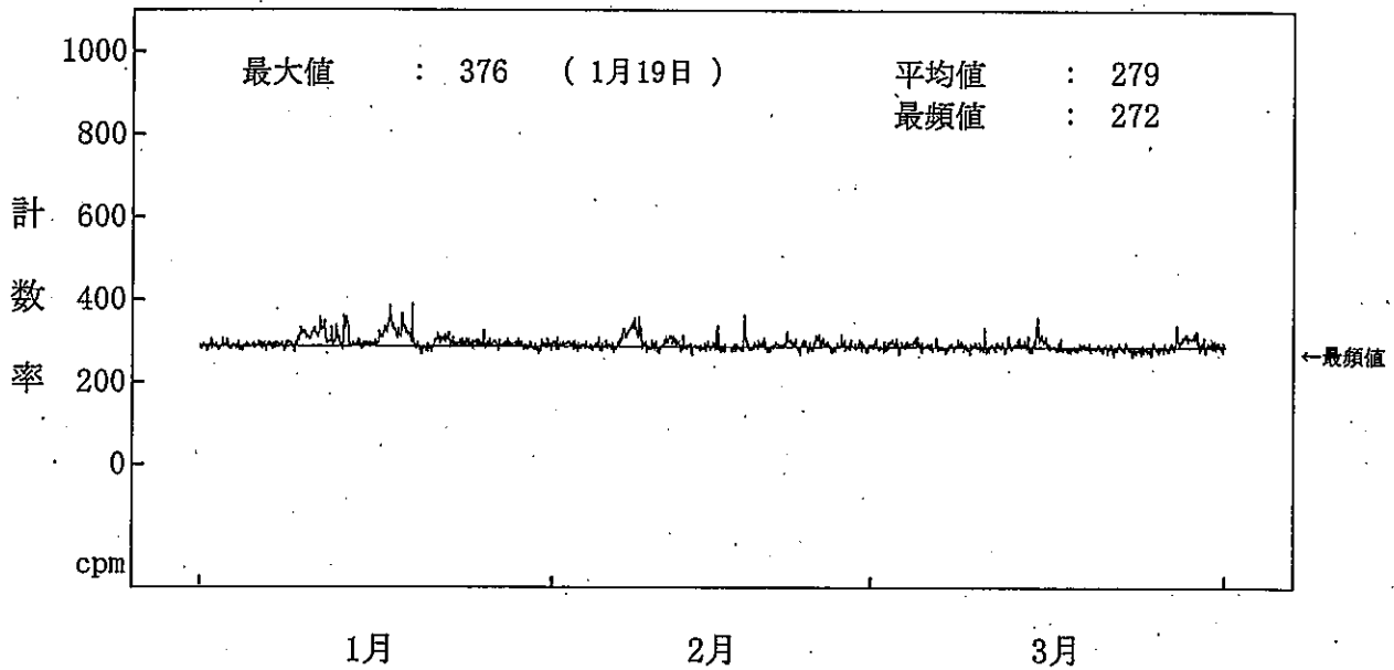
図一 2 - 8 海水(放水)中の全ガンマ線計数率監視結果(1号機放水口モニター(A)) (注) 2月16日の欠測は、停電作業によるものである。
