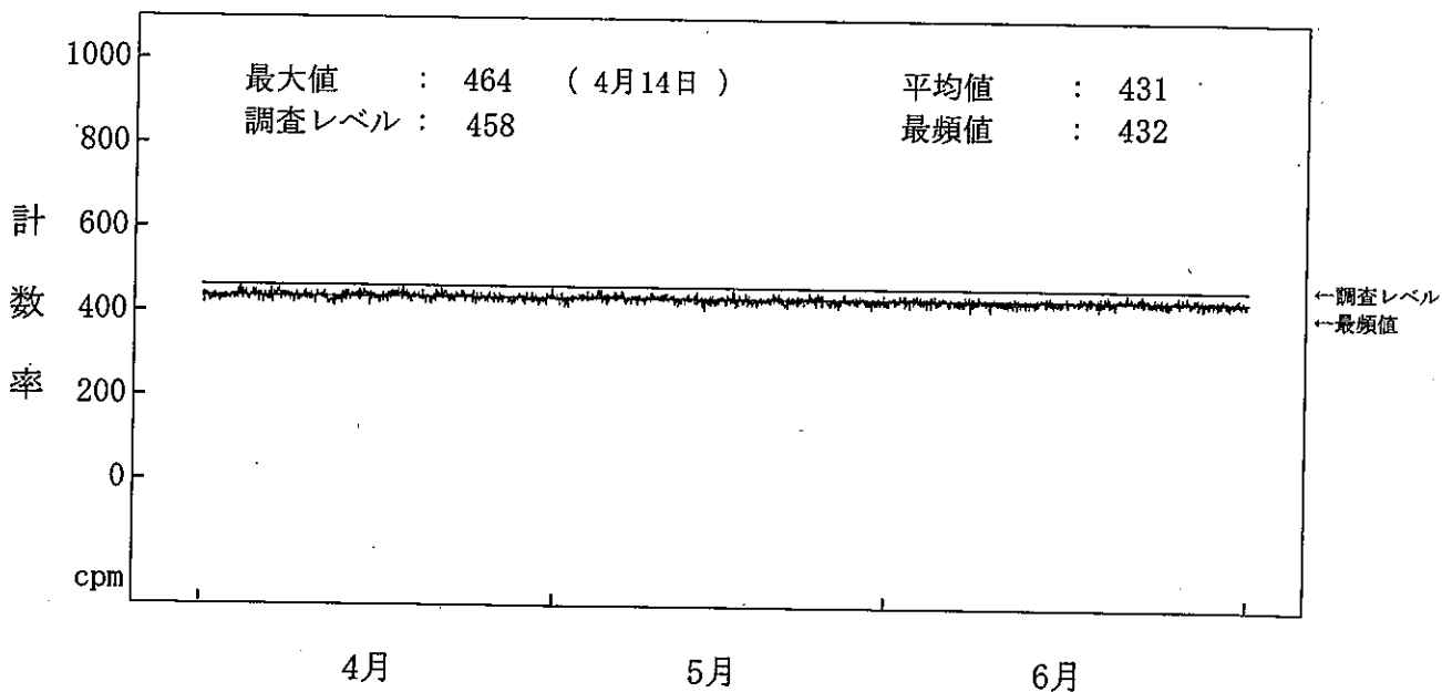
図一 2 - 1 0 海水(放水)中の全ガンマ線計数率監視結果(2号機放水口モニター) (注) 4月27日、5月25日、6月15日の欠測は、定期点検によるものである。
