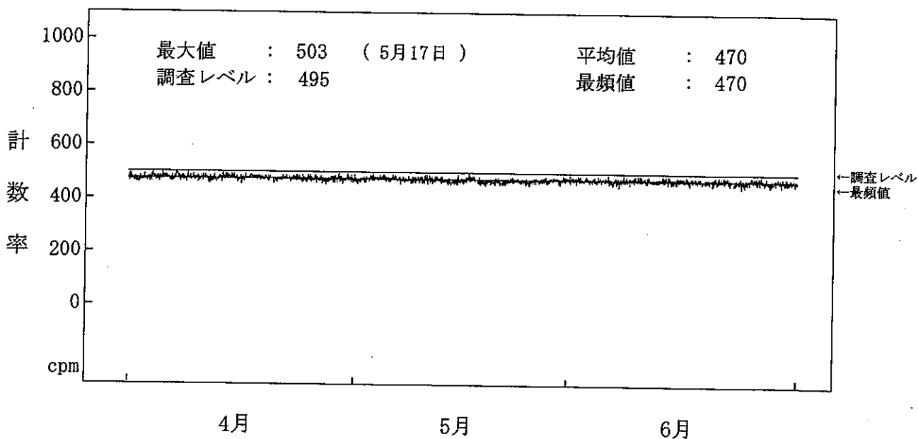
図一 2 - 1 1 海水(放水)中の全ガンマ線計数率監視結果(3号機放水口モニター) (注) 4月20日、5月18日、6月22日の欠測は、定期点検によるものである。
