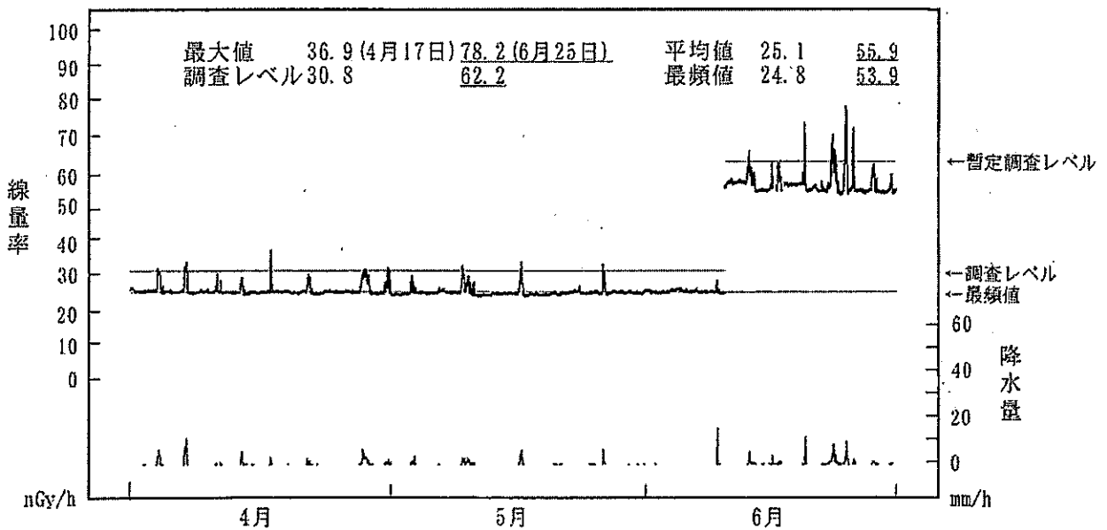
図-2-2 空間ガンマ線線量率監視結果 (小屋取局)
