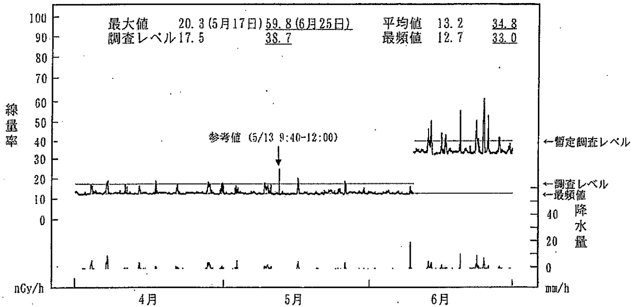
図-2-1 空間ガンマ線線量率監視結果 (女川局)
