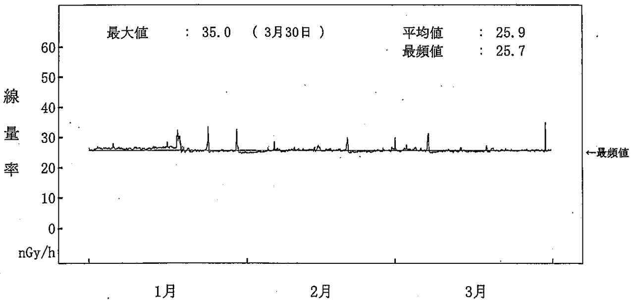
図-2-7 空間ガンマ線線量率監視結果 (前網局) (注) 下方を鉛で遮へいたNaI (T1) 検出器により測定した。
