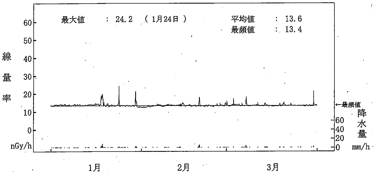
図-2-5 空間ガンマ線線量率監視結果 (寺間局)
