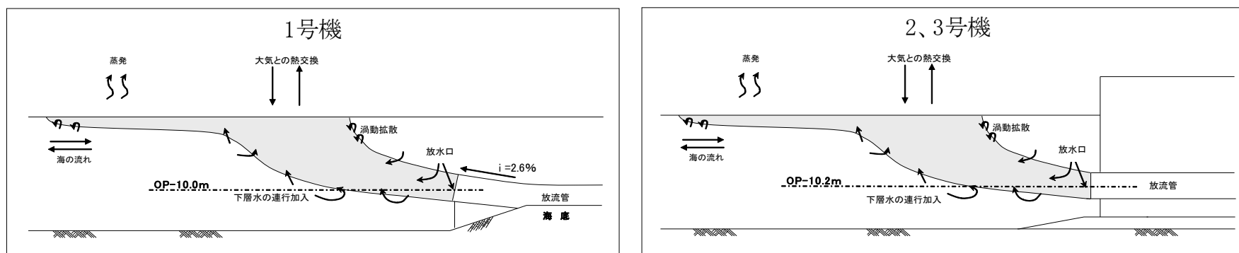
図-3-(2) 水中放流方式における温排水の拡散概念
