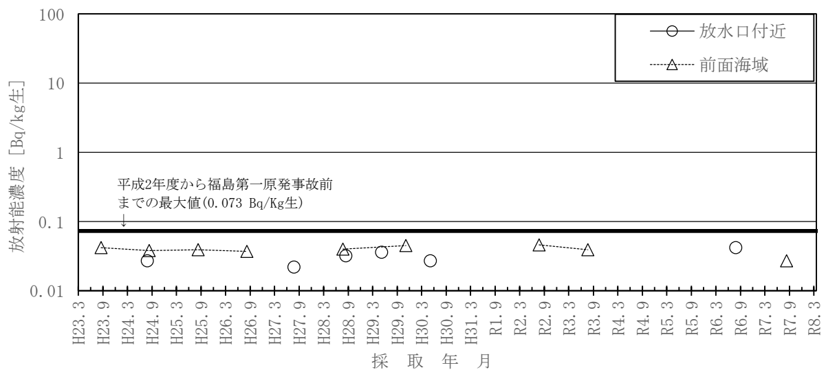
図－２７ アラメのSr-90濃度の推移
