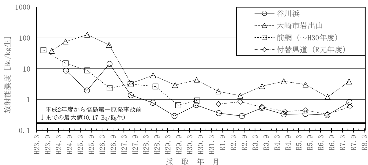
図－10 ヨモギのCs-137濃度の推移
