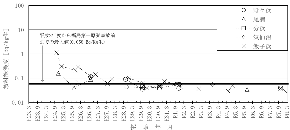
図－１３ マガキのCs-137濃度の推移
