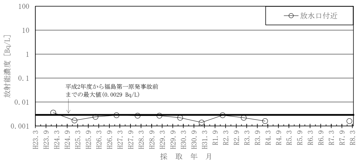
図－２６ 海水のSr-90濃度の推移
