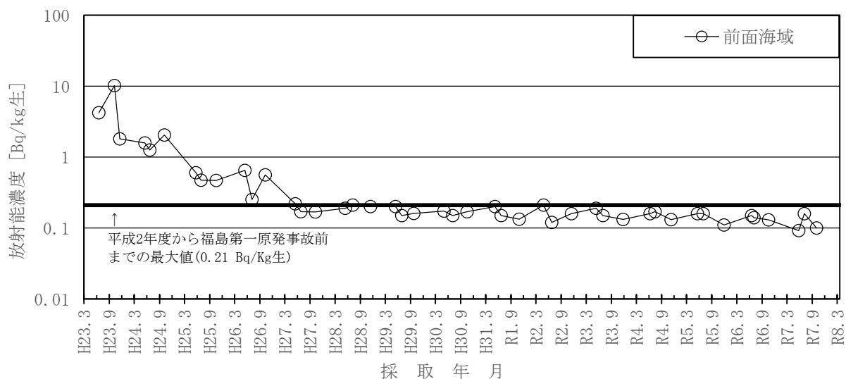
図－１２ アイナメのCs-137濃度の推移
