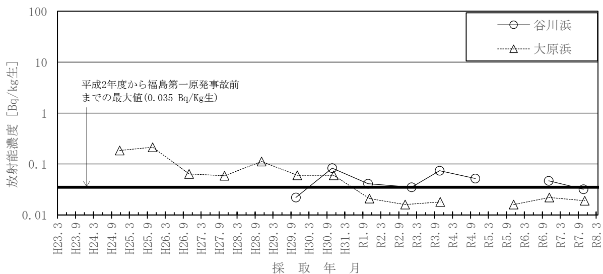
図－6 精米のCs-137濃度の推移
