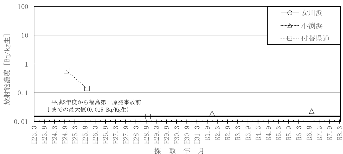
図－8 大根（根）のCs-137濃度の推移
