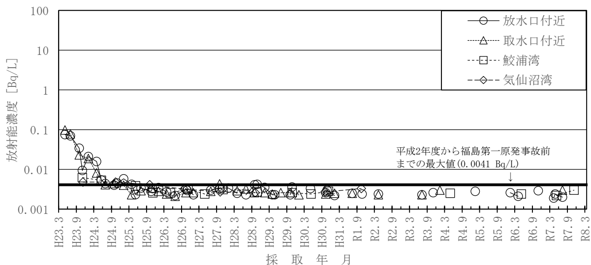
図－１８ 海水のCs-137濃度の推移
