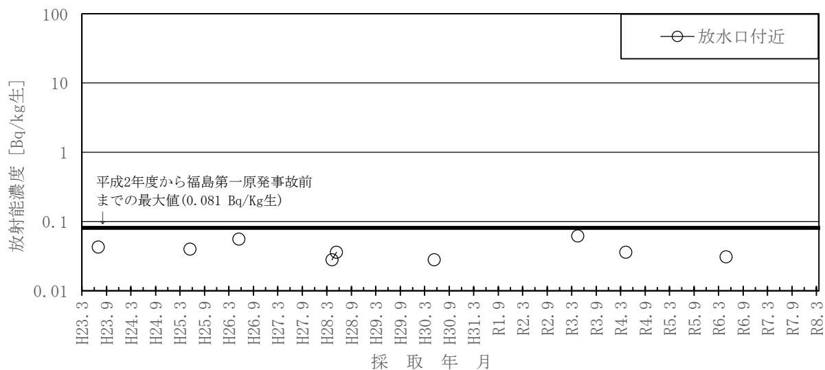
図－2 5 ワカメのSr-90濃度の推移
