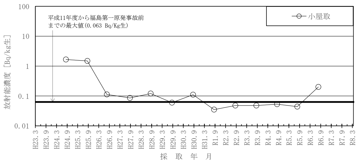
図-16 キタムラサキウニのCs-137濃度の推移
