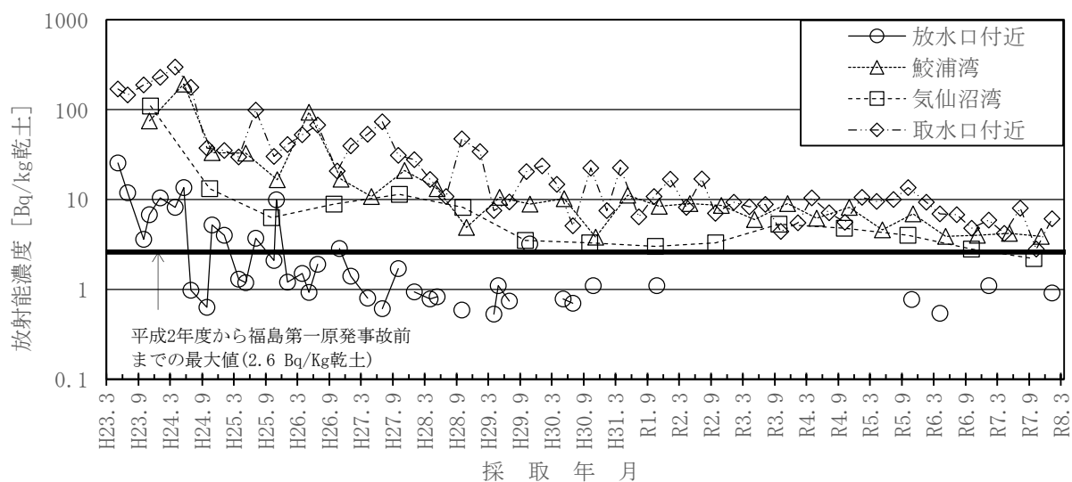
図－１９ 海底土のCs-137濃度の推移
