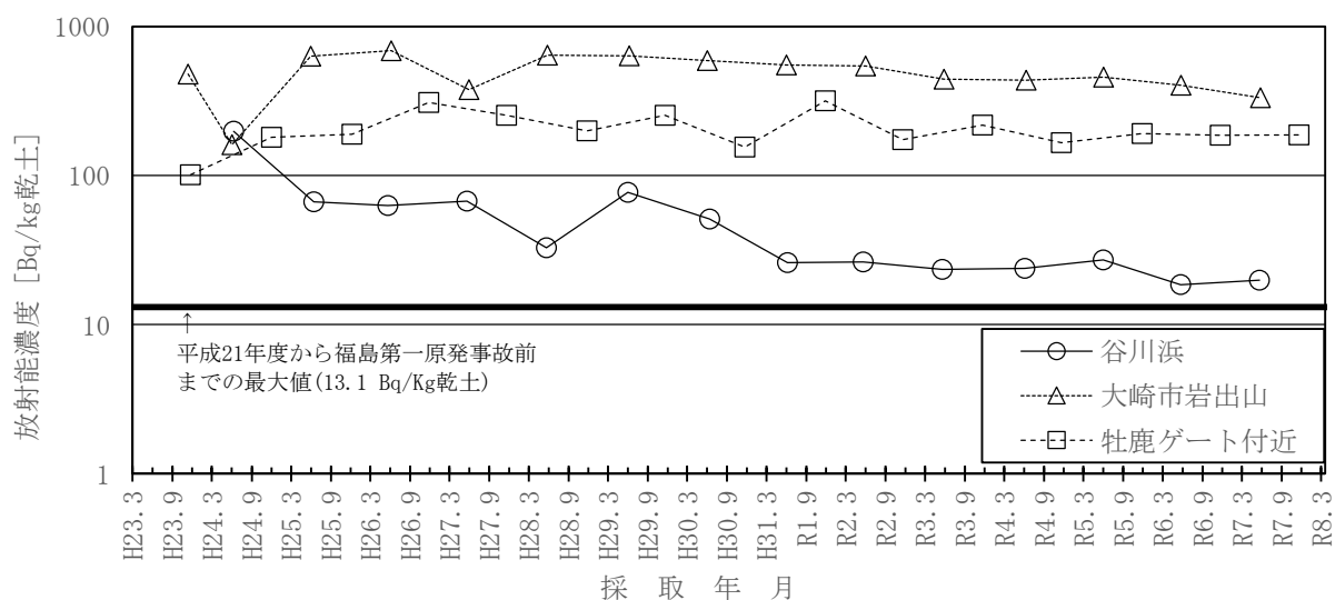
図－9 陸土のCs-137濃度の推移
