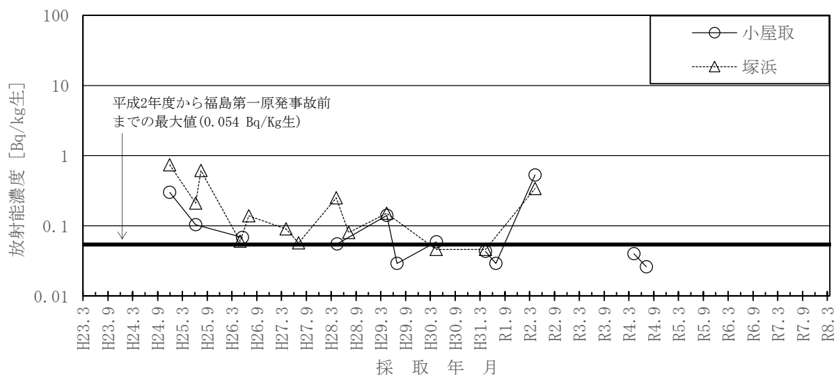
図-14 マボヤのCs-137濃度の推移
