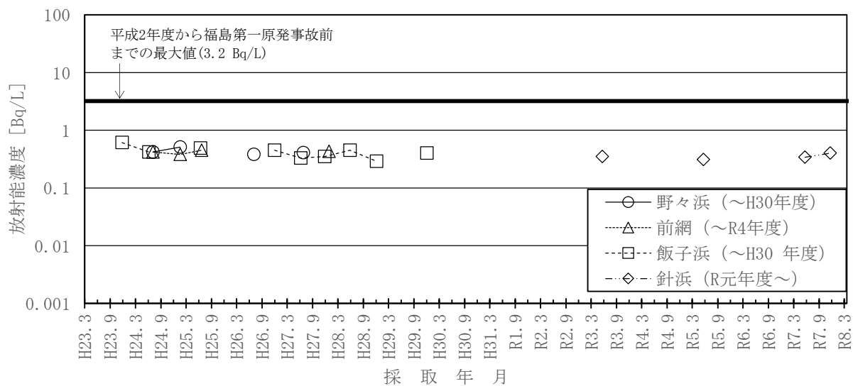
図－２８ 陸水のH-3濃度の推移
