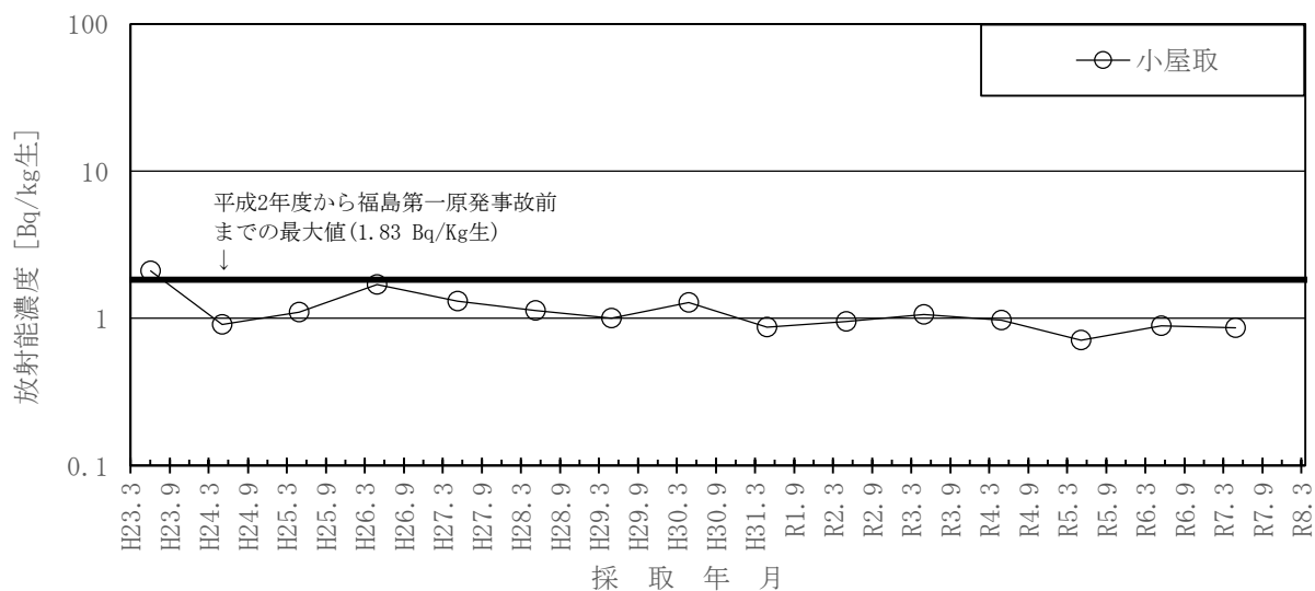
図－2 4 松葉のSr-90濃度の推移
