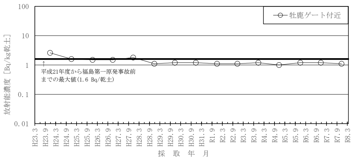
図－２２ 陸土のSr-90濃度の推移
