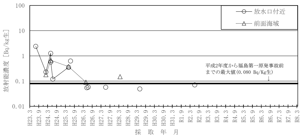
図－１７ ワカメのCs-137濃度の推移
