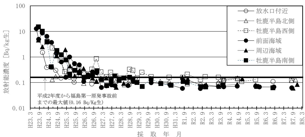
図－２０ アラメのCs-137濃度の推移
