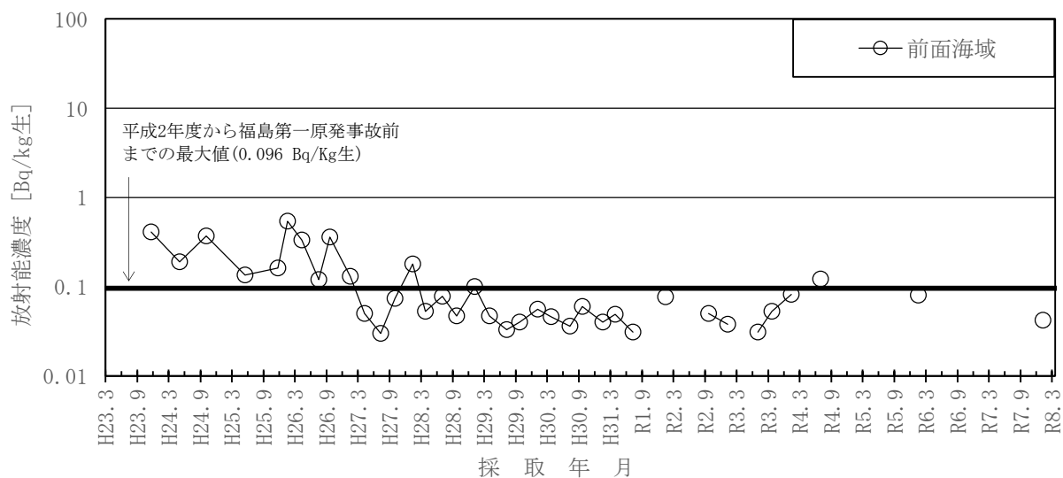
図－２１ ムラサキイガイのCs-137濃度の推移
