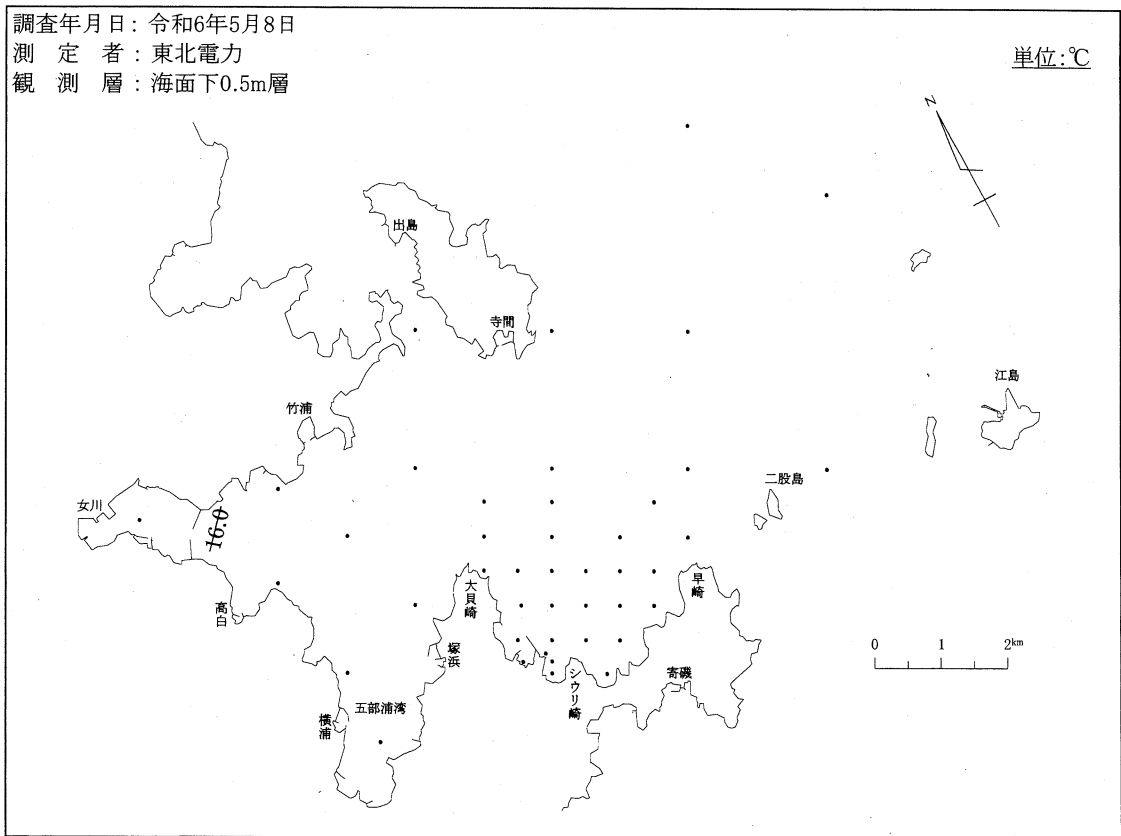
図-4-(2) 等温線
