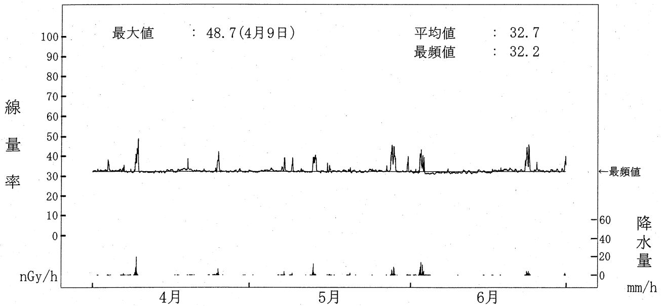
図-2-10 NaI(Tl)検出器による空間ガンマ線量率監視結果 (江島局) (注) 6月14日の欠測は、定期点検によるものである。
