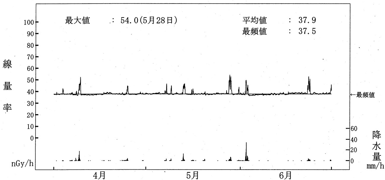
図-2-9 NaI(Tl)検出器による空間ガンマ線量率監視結果(寺間局) (注) 6月24日の欠測は、定期点検によるものである。
