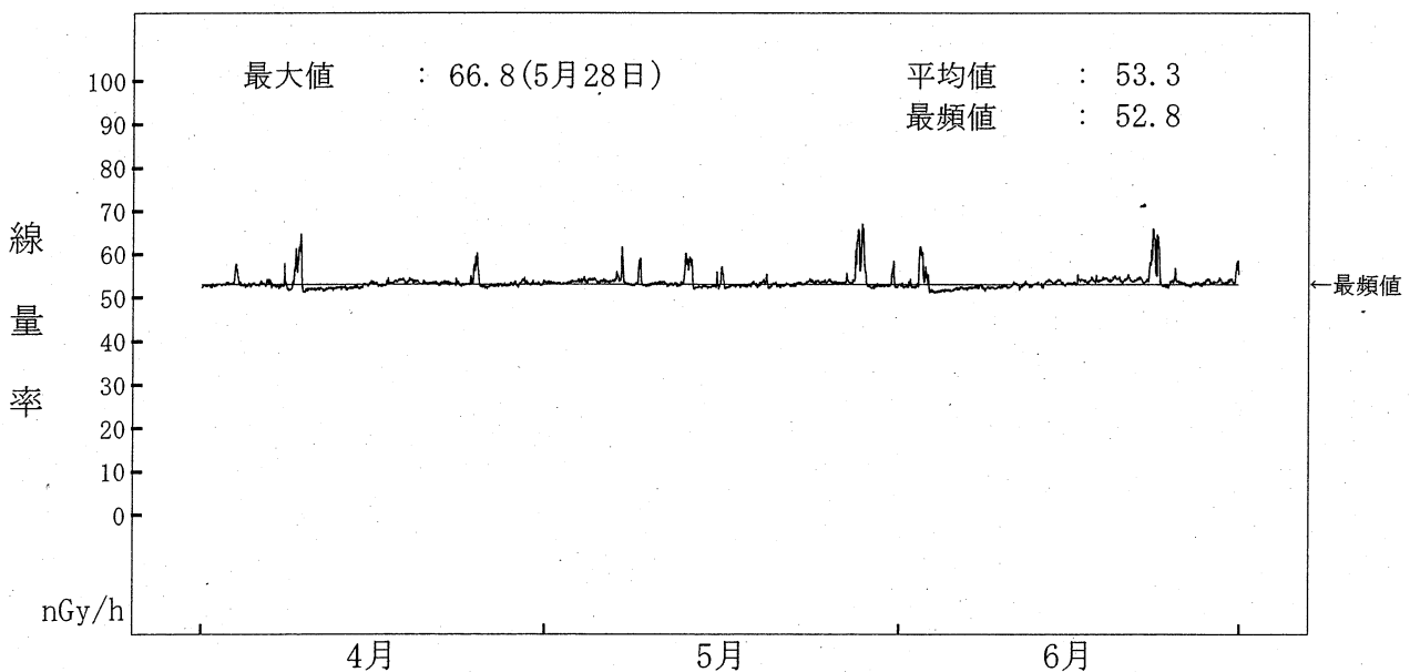
図-2-11 NaI(Tl)検出器による空間ガンマ線量率監視結果 (前網局) (注) 6月13日の欠測は、定期点検によるものである。
