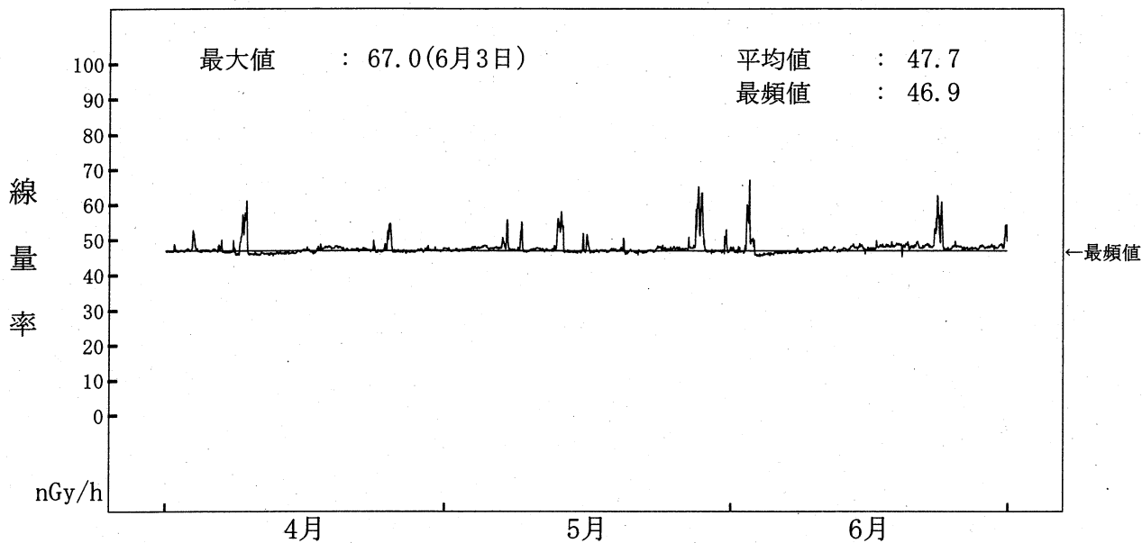
図-2-8 NaI(Tl)検出器による空間ガンマ線量率監視結果(塚浜局) (注) 6月12日の欠測は、定期点検によるものである。
