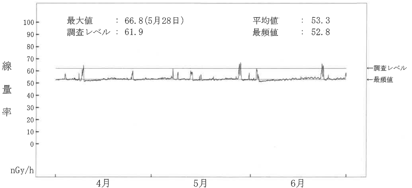
図-2-11 NaI(Tl)検出器による空間ガンマ線量率監視結果 (前網局) (注) 6月13日の欠測は、定期点検によるものである。
