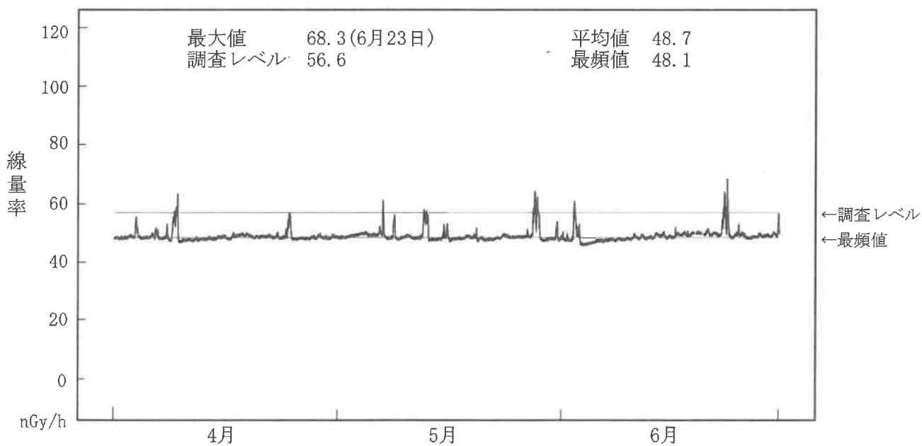
図-2-6 NaI(Tl)検出器による空間ガンマ線量率監視結果（谷川局）
