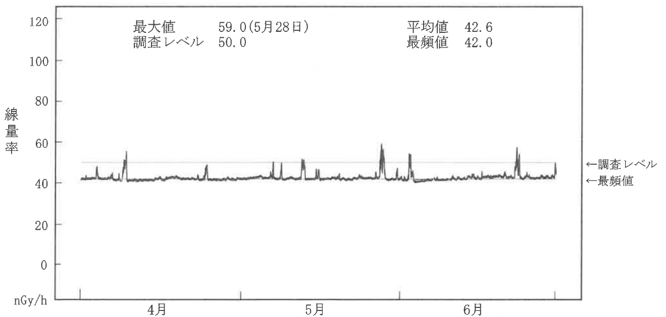
図-2-2 NaI(Tl)検出器による空間ガンマ線量率監視結果（飯子浜局）
