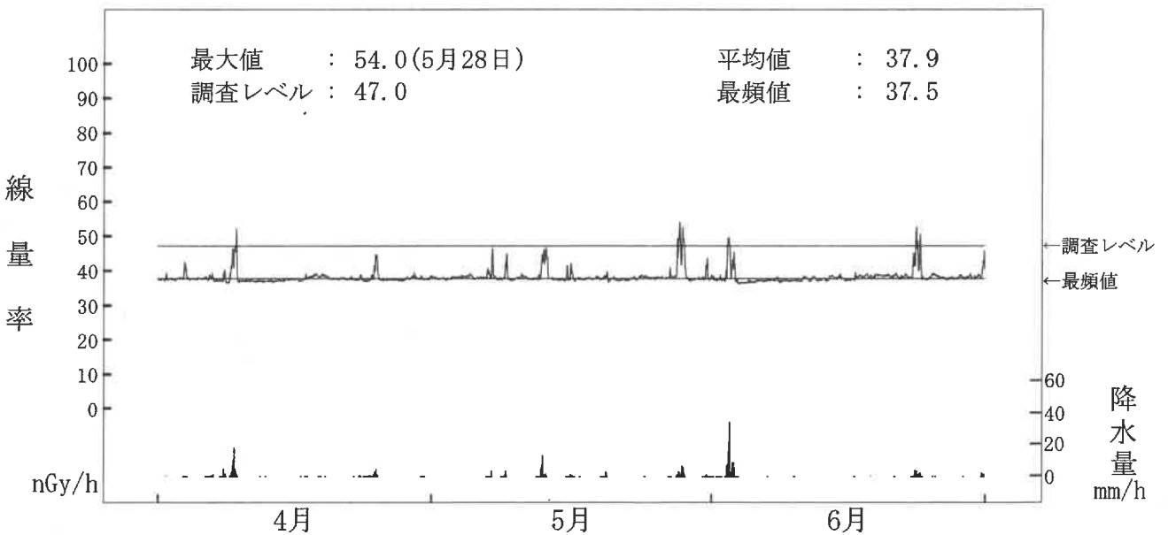
図-2-9 NaI(Tl)検出器による空間ガンマ線量率監視結果 (寺間局) (注) 6月24日の欠測は、定期点検によるものである。
