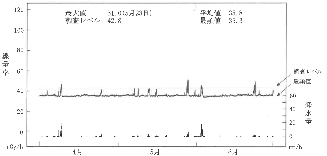
図-2-4 NaI(Tl)検出器による空間ガンマ線量率監視結果 (寄磯局)
