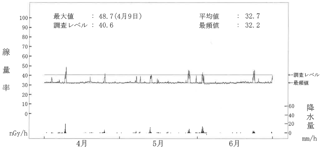
図-2-10 NaI(Tl)検出器による空間ガンマ線量率監視結果 (江島局) (注) 6月14日の欠測は、定期点検によるものである。
