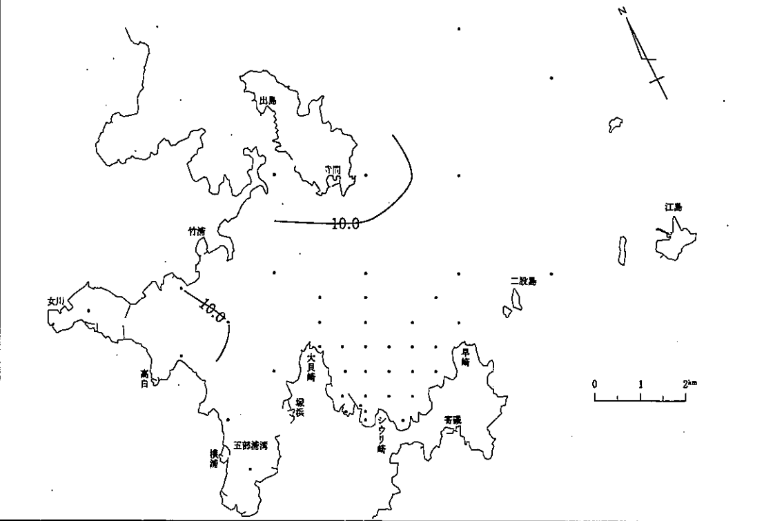
図-4-(2) 等温線
