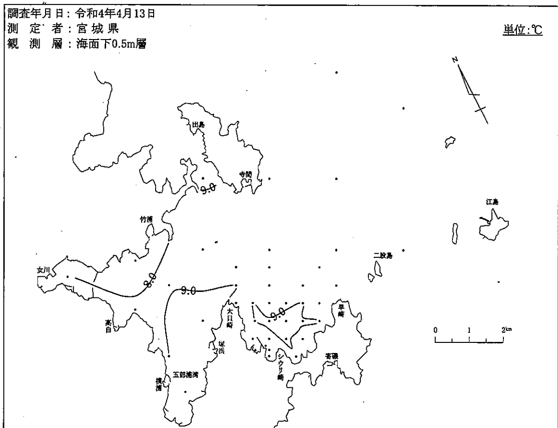
図-2-(2) 等温線
