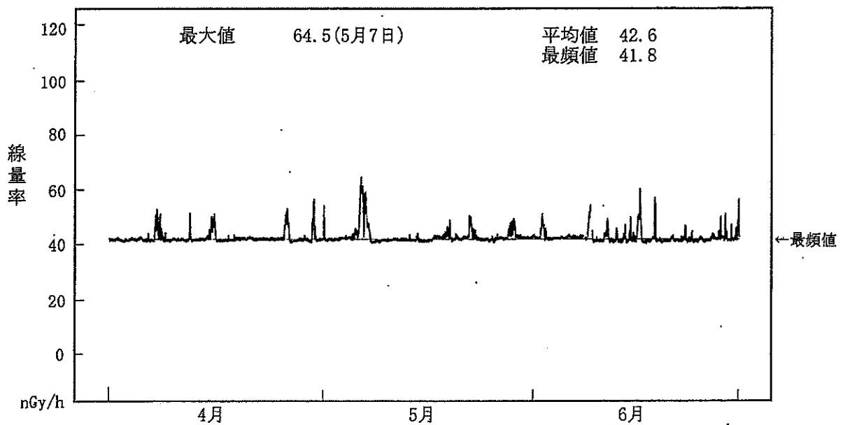
図一2-2 NaI(Tl)検出器による空間ガンマ線量率監視結果（飯子浜局）
