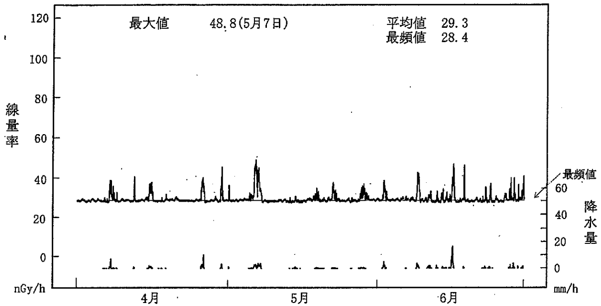
図一2-1 NaI(Tl)検出器による空間ガンマ線量率監視結果（女川局）
