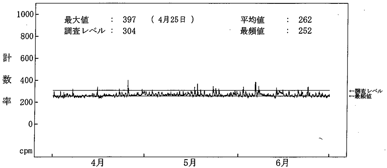
図-2-13 海水(放水)中の全ガンマ線計数率監視結果(1号機放水口モニター(B)) (注) 6月1日の欠測は、定期点検によるものである。
