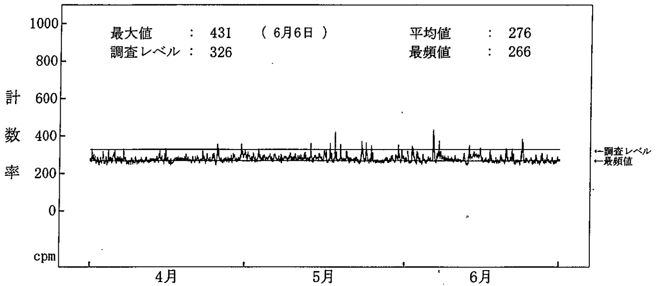
図-2-12 海水(放水)中の全ガンマ線計数率監視結果(1号機放水口モニター(A)) (注) 6月1日の欠測は、定期点検によるものである。
