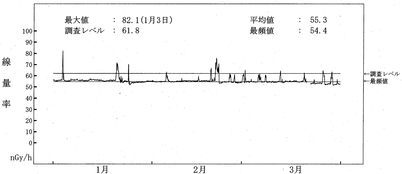
図-2-11 NaI(Tl)検出器による空間ガンマ線量率監視結果(前網局) (注) 3月21日~22日の欠測は、機器更新によるものである。
