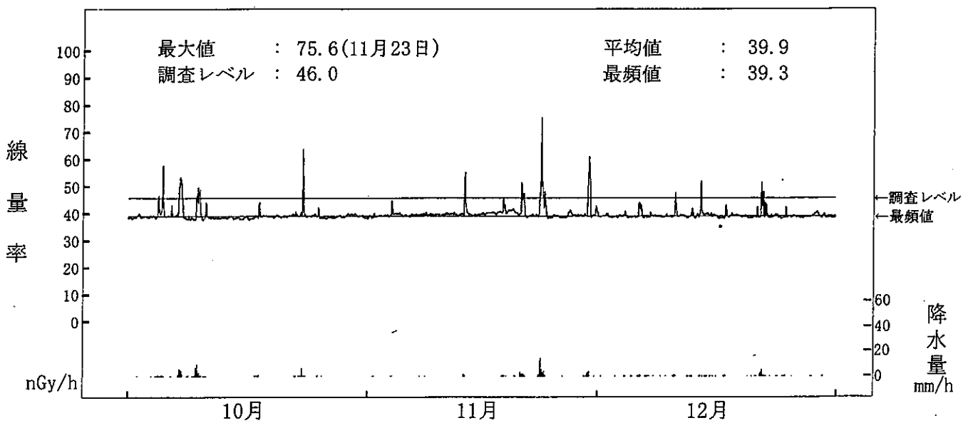
図-2-9 空間ガンマ線量率監視結果 (寺間局)
