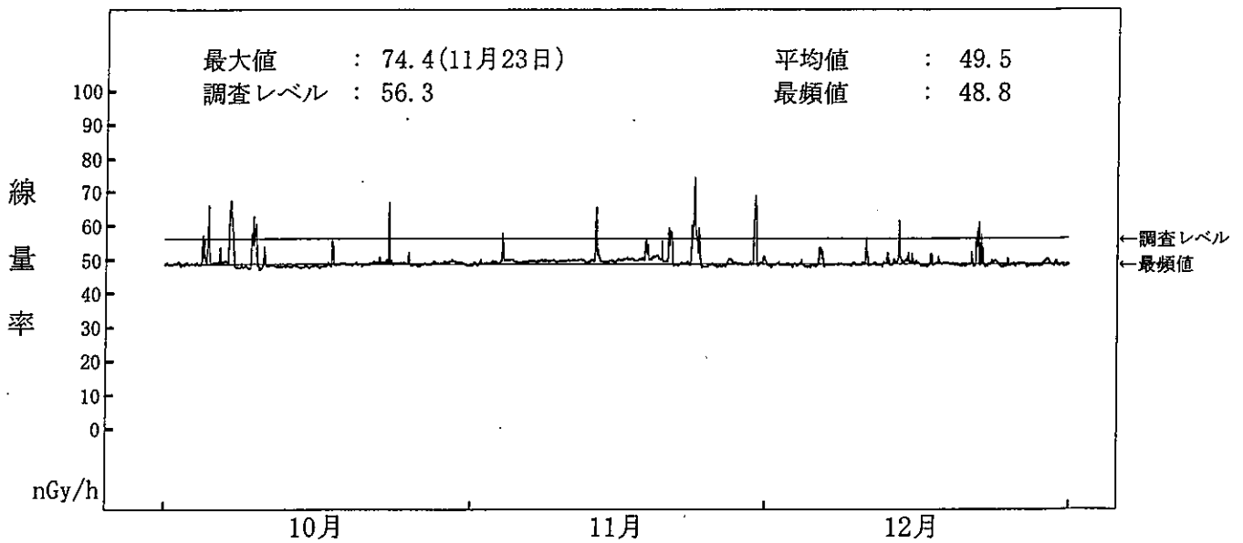
図-2-8 空間ガンマ線量率監視結果 (塚浜局)
