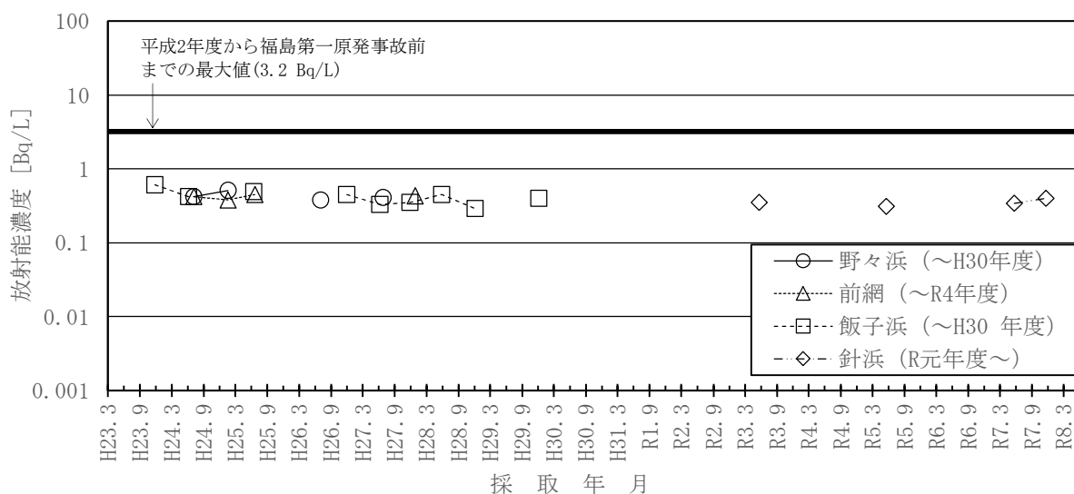
図－２－３２ 陸水のH-3濃度の推移
