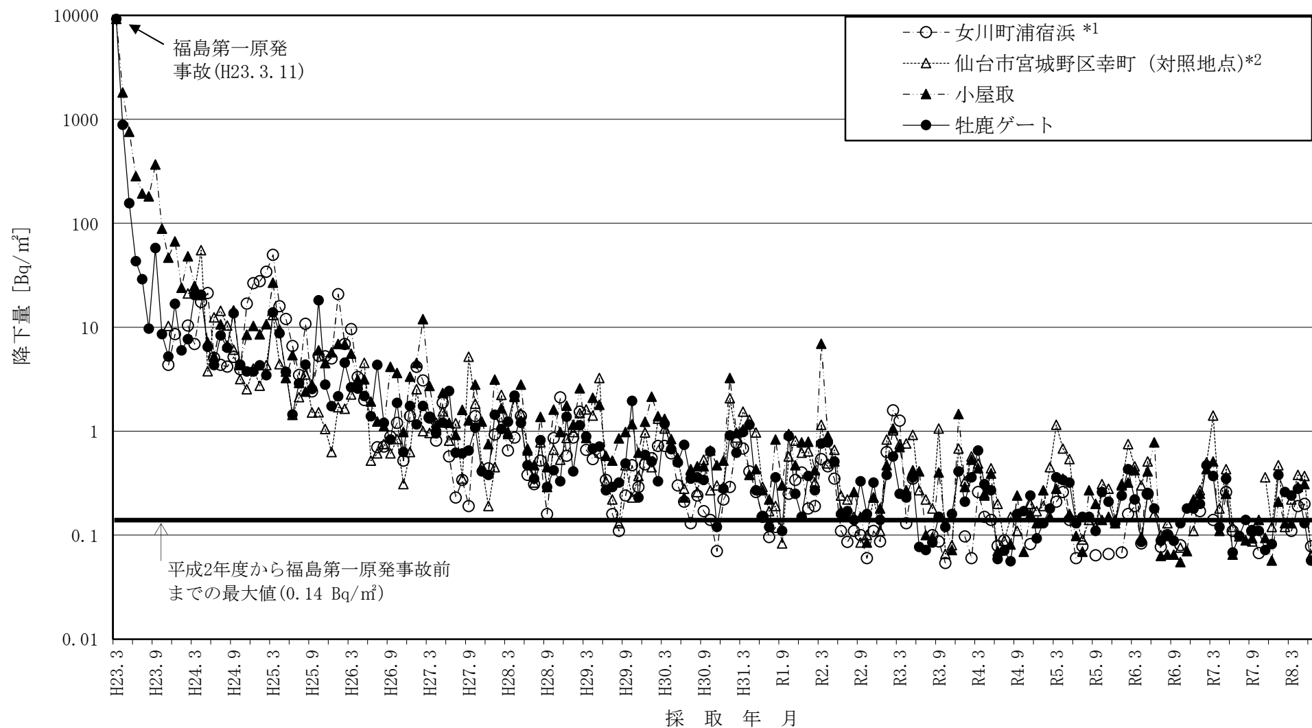
図-2-20 福島第一原発事故後のCs-137の月間降下量の推移
