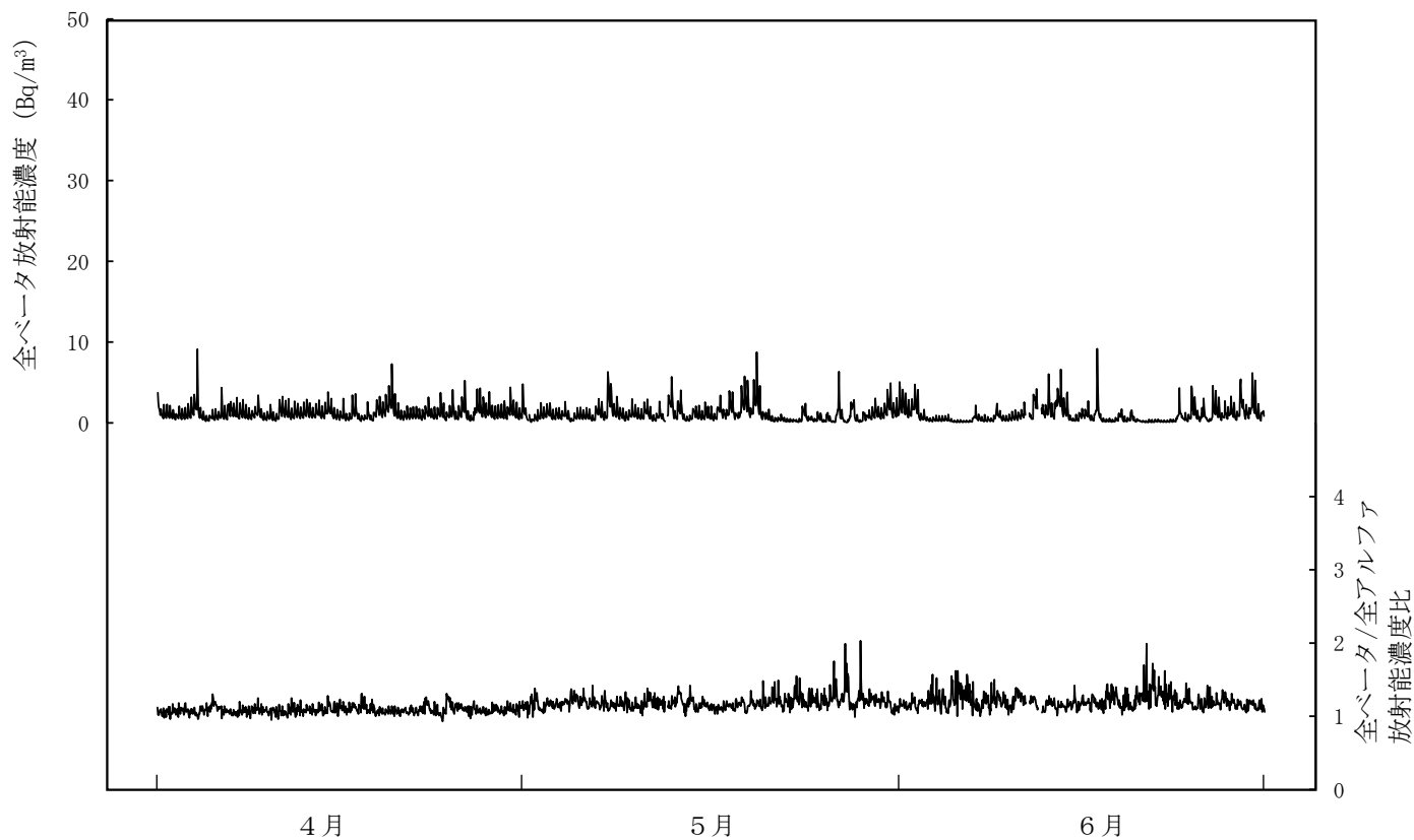
図－２－１７ 大気中の放射性物質の全ベータ放射能濃度及び 全ベータ／全アルファ放射能濃度比（鮫浦局）
