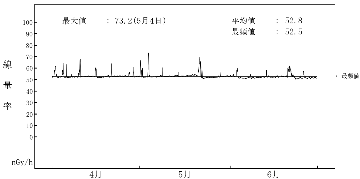
図－２－１１ NaI(Tl)検出器による空間ガンマ線量率監視結果（前網局）
