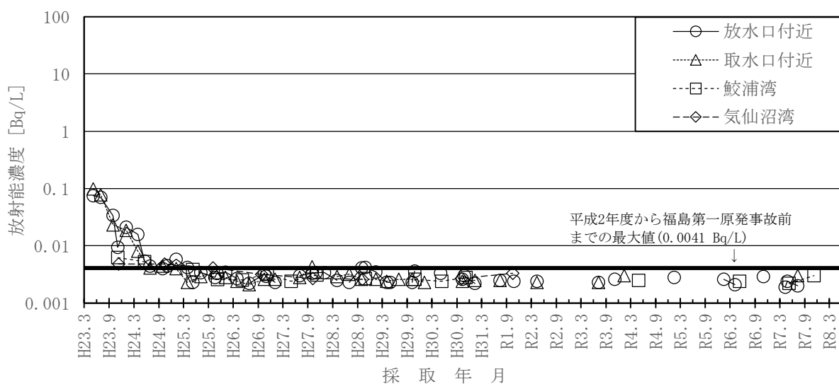
図-2-27 海水のCs-137濃度の推移
