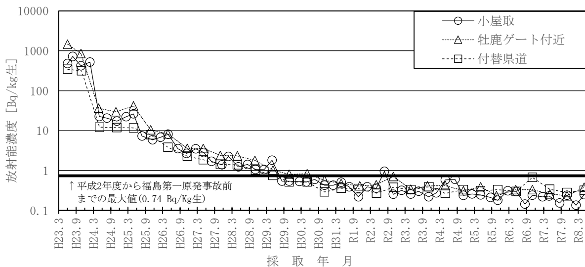
図－２－２３ 松葉のCs-137濃度の推移
