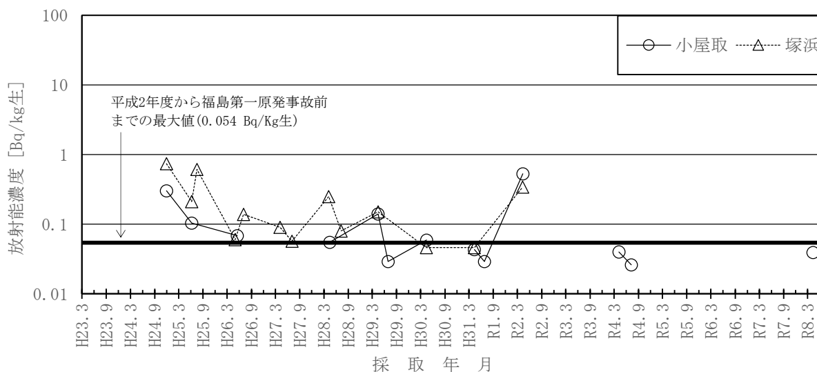
図-2-25 マボヤのCs-137濃度の推移
