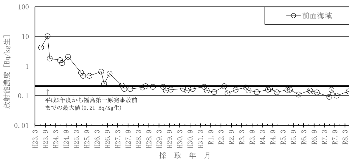
図－２－２４ アイナメのCs-137濃度の推移
