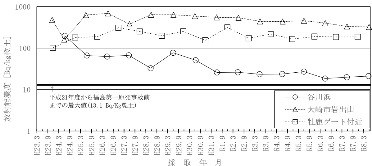
図－２－２２ 陸土のCs-137濃度の推移
