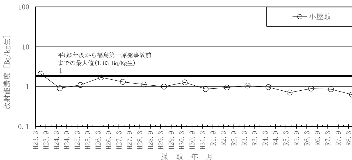
図－２－３０ 松葉のSr-90濃度の推移
