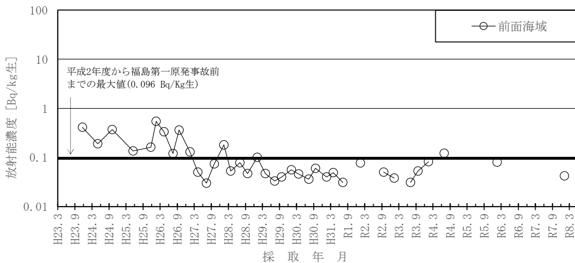
図－２－２９ ムラサキイガイのCs-137濃度の推移
