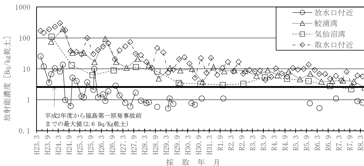
図－２－２８ 海底土のCs-137濃度の推移
