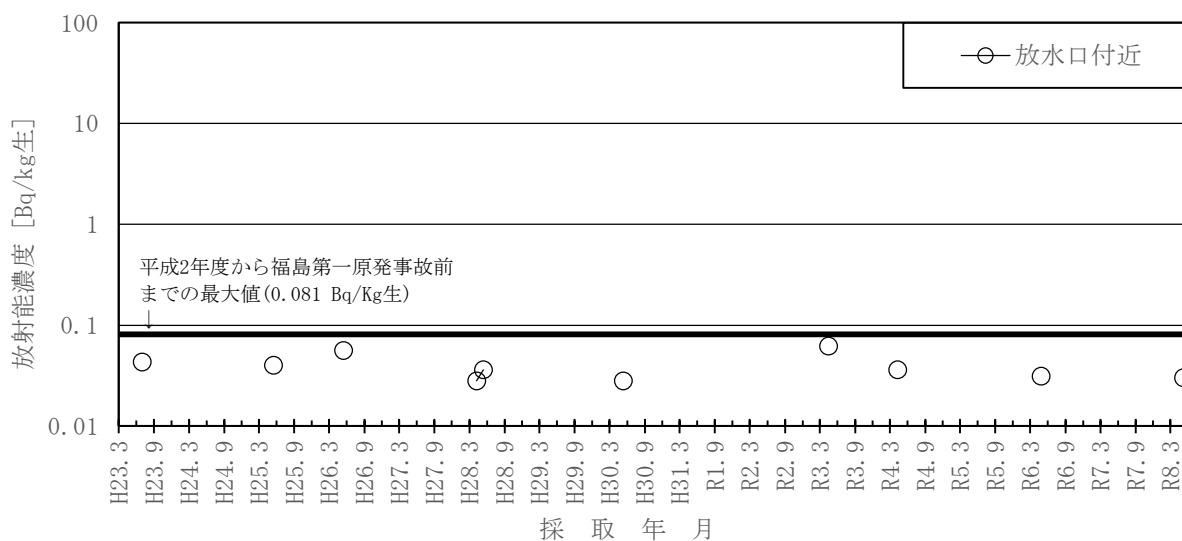
図－２－３１ ワカメのSr-90濃度の推移
