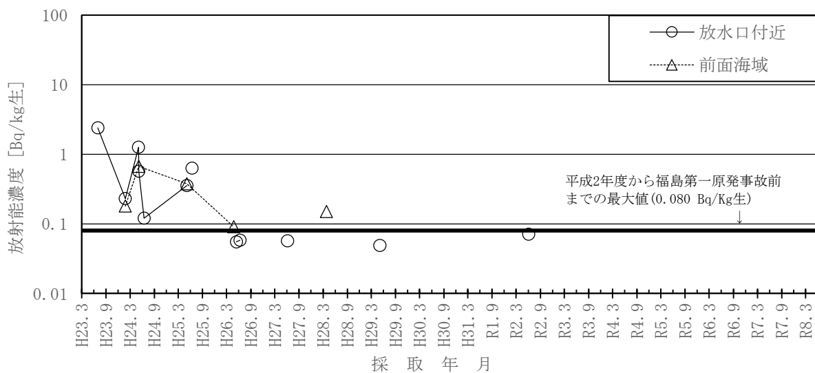
図-2-26 ワカメのCs-137濃度の推移
