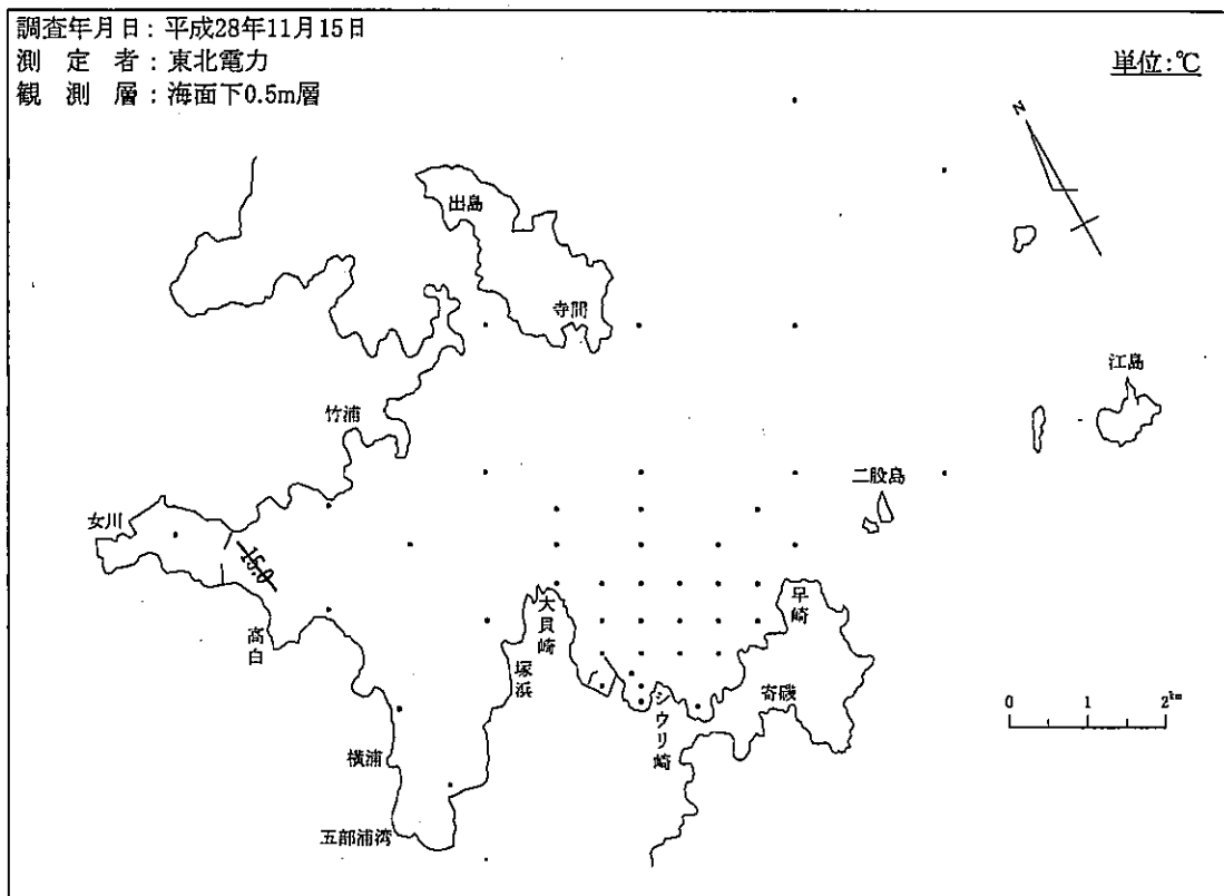
図-4-(2) 等温線
