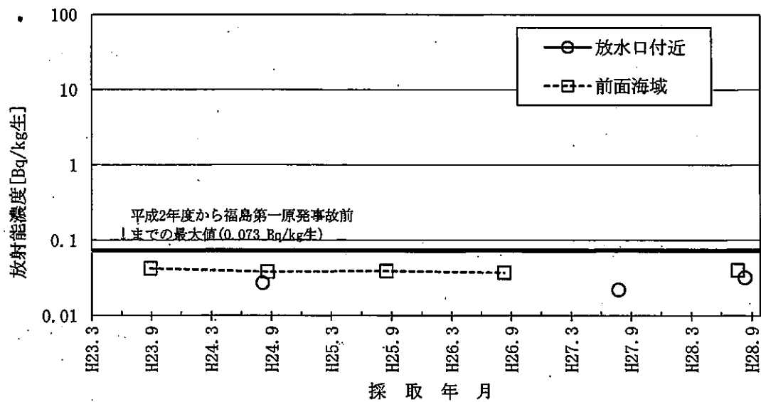
図-2-26 アラメのSr-90濃度の推移
