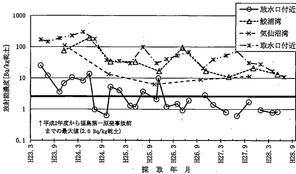
図-2-2-2 海底土のCs-137濃度の推移
