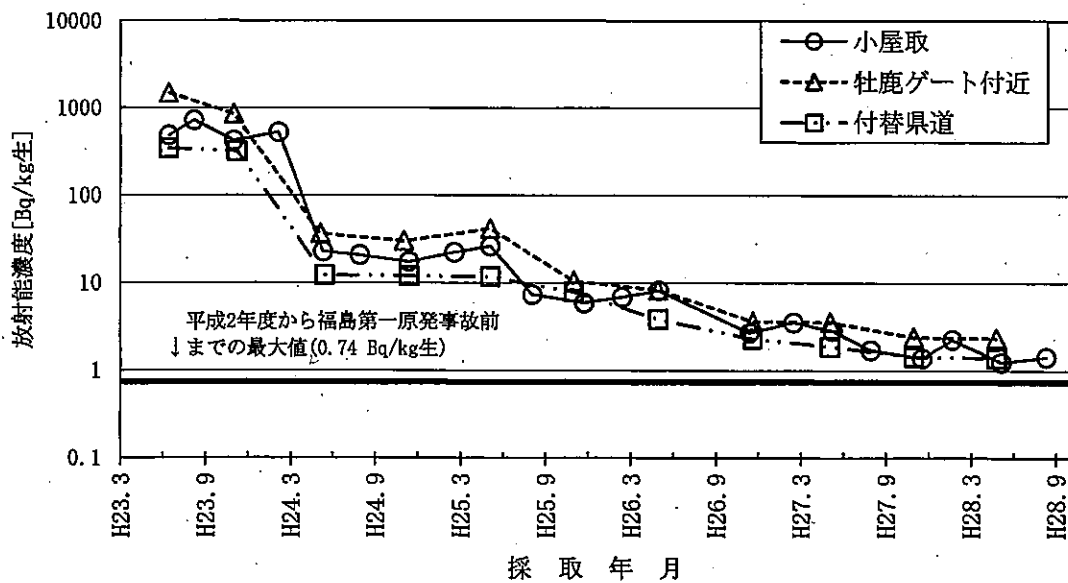
図-2-17 松葉のCs-137濃度の推移
