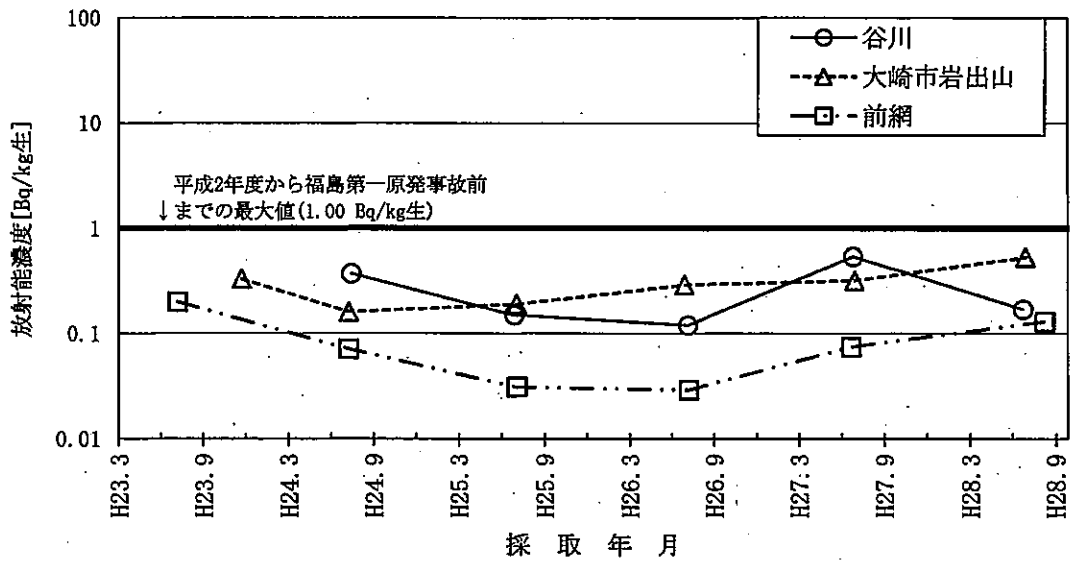
図-2-25 ヨモギのSr-90濃度の推移
