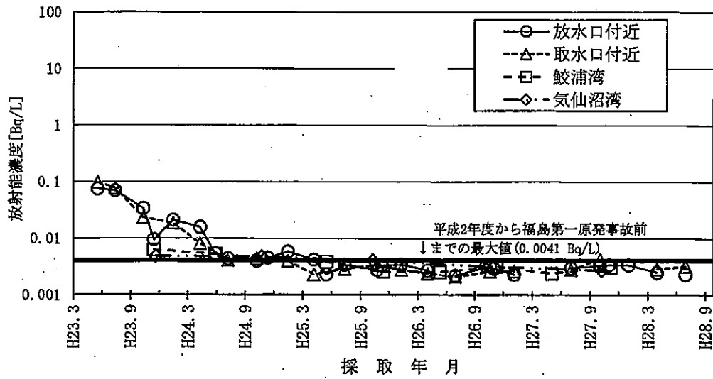
図-2-2-1 海水のCs-137濃度の推移
