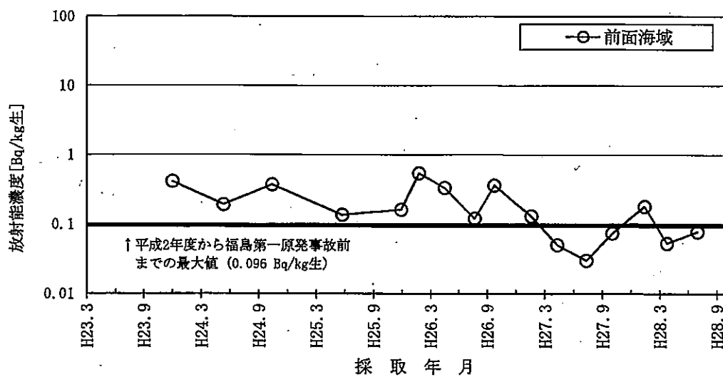
図-2-2-3 ムラサキガイのCs-137濃度の推移
