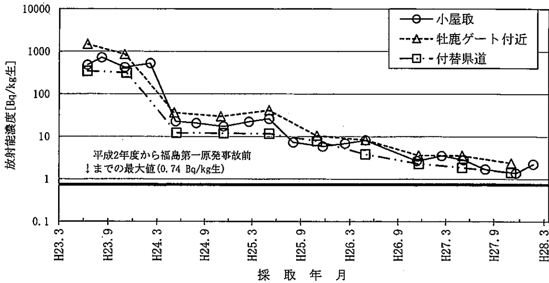
図-11 松葉のCs-137濃度の推移
