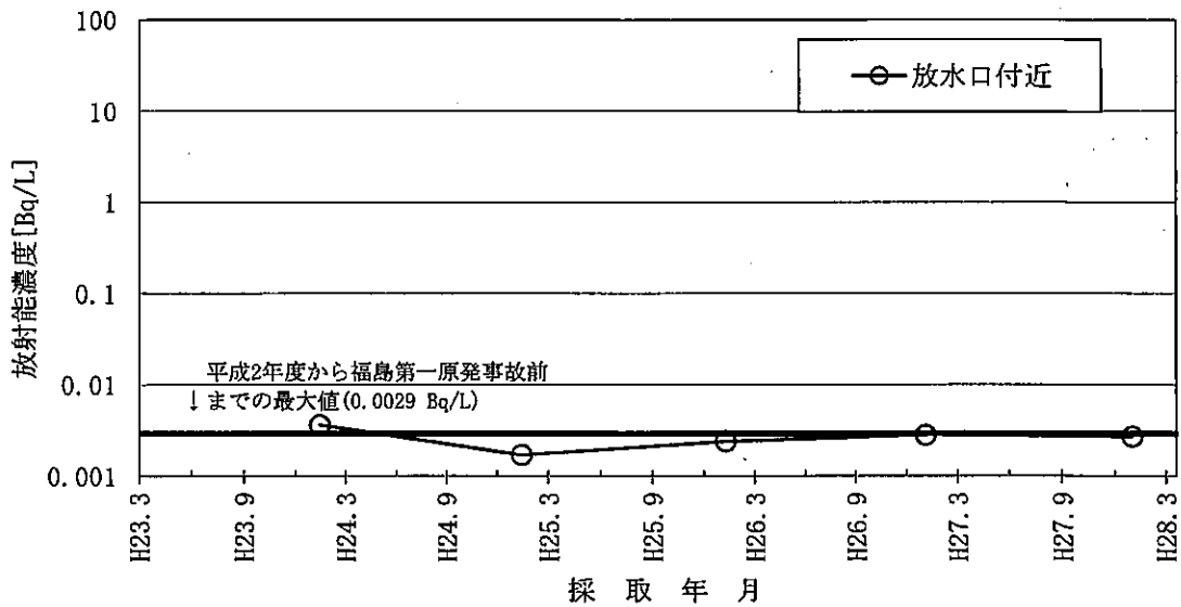
図-27 海水のSr-90濃度の推移
