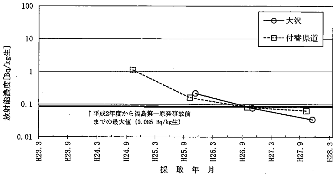
図-8 大根（葉）のCs-137濃度の推移
