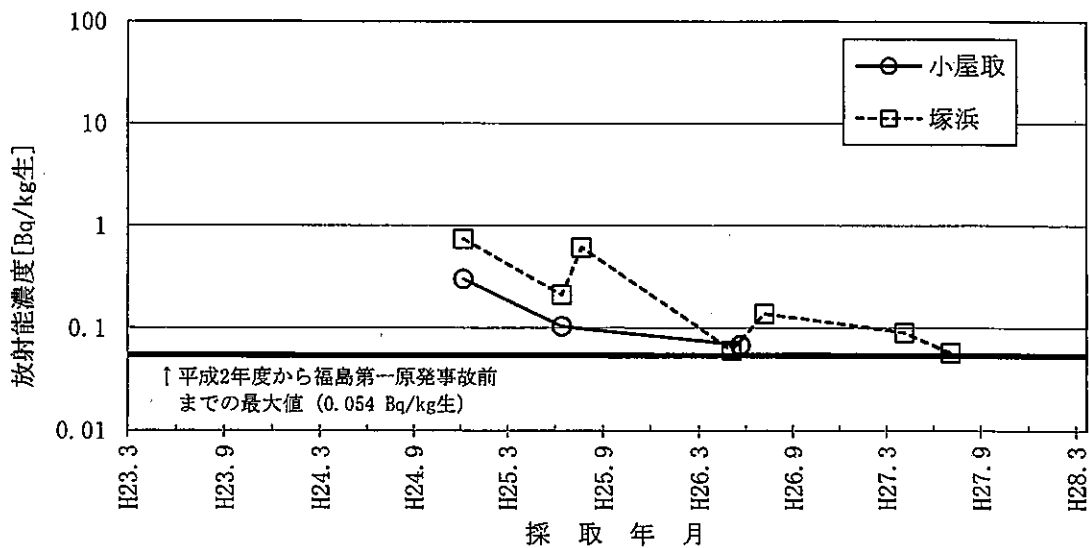
図-13 ホヤのCs-137濃度の推移
