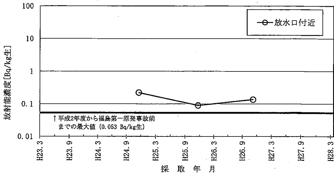
図-14 アワビのCs-137濃度の推移
