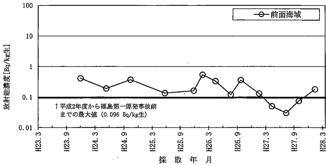
図-21 ムラサキガイのCs-137濃度の推移
