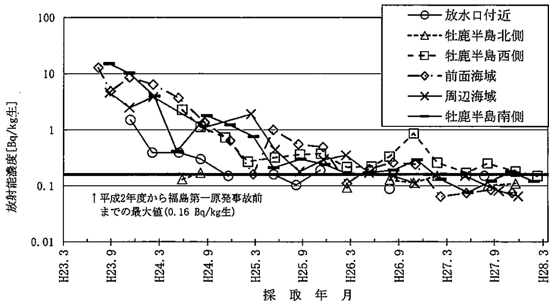
図-20 アラメのCs-137濃度の推移
