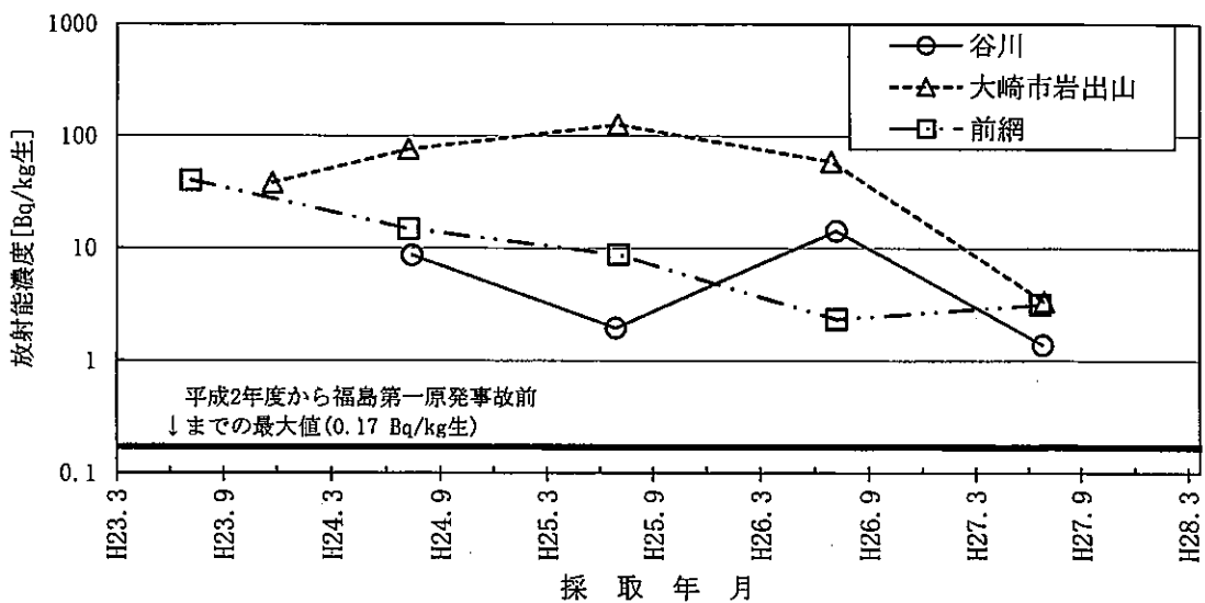
図-10 ヨモギのCs-137濃度の推移
