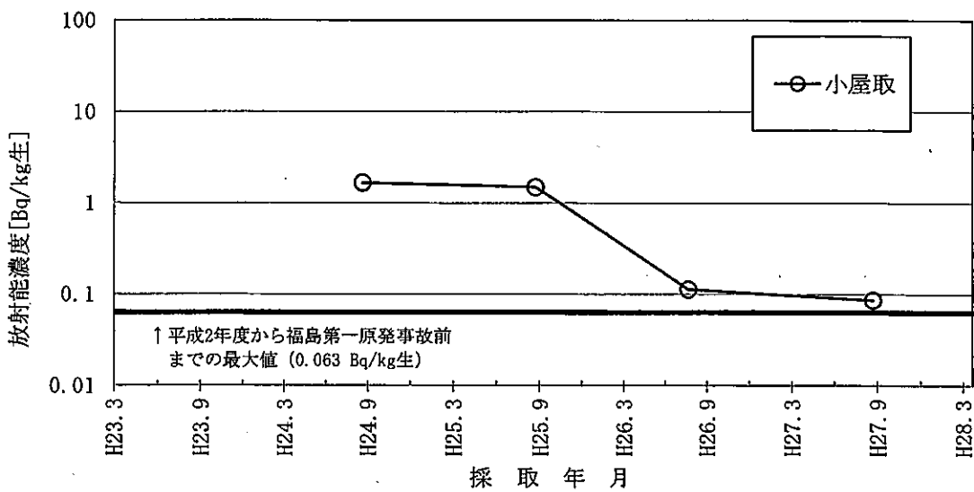
図-15 ウニのCs-137濃度の推移
