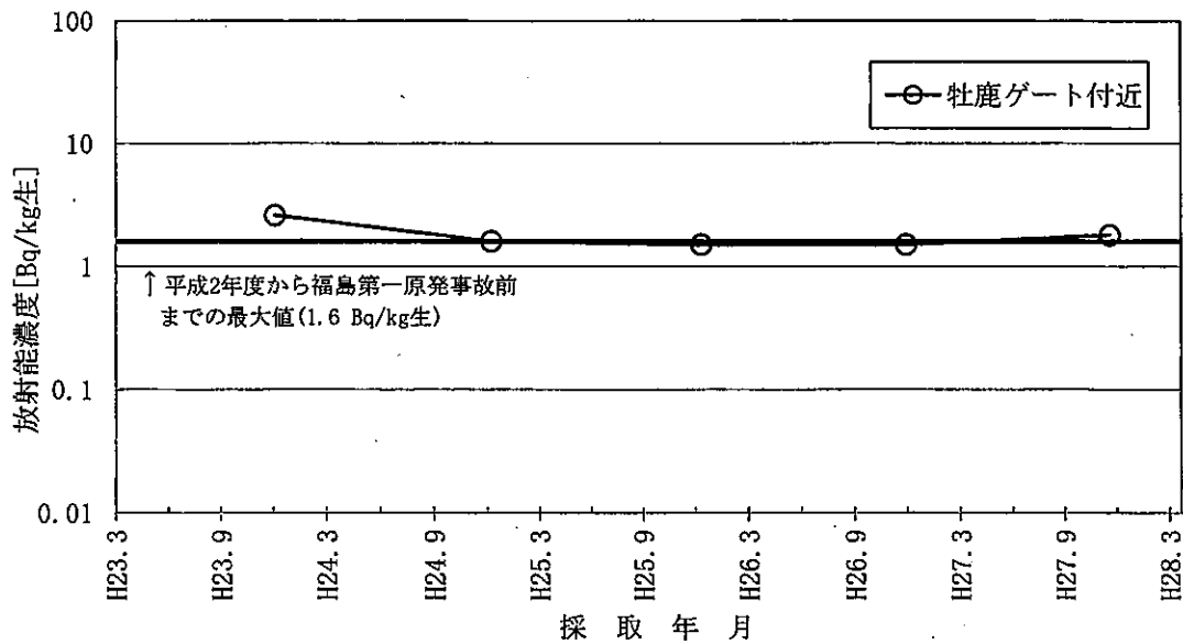
図-22 陸土のSr-90濃度の推移
