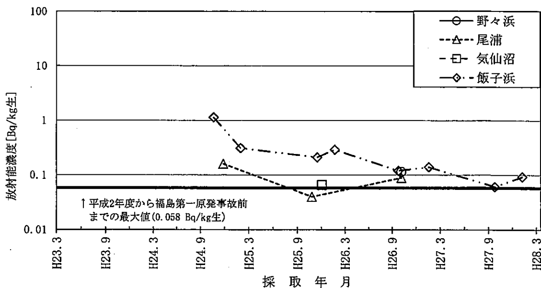
図-16 カキのCs-137濃度の推移
