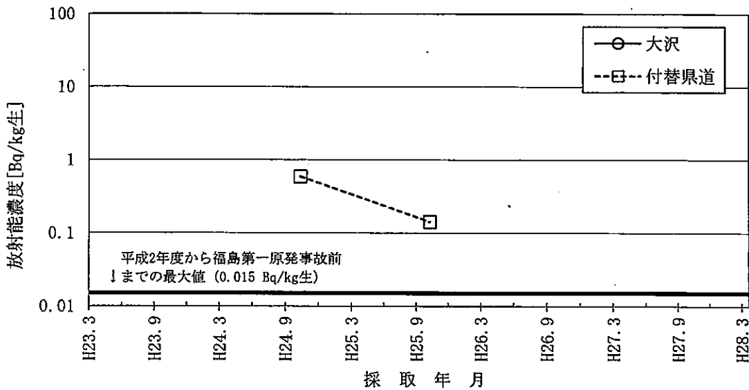
図-7 大根（根）のCs-137濃度の推移
