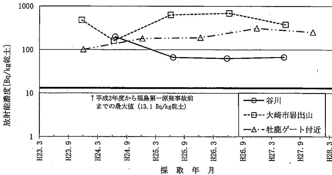
図-9 陸土のCs-137濃度の推移
