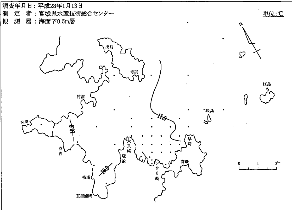
図-2-1(2) 等温線
