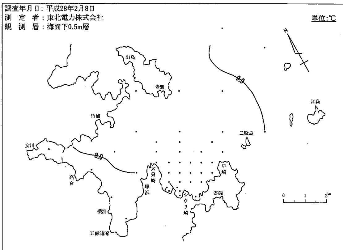
図-4-(2) 等温線
