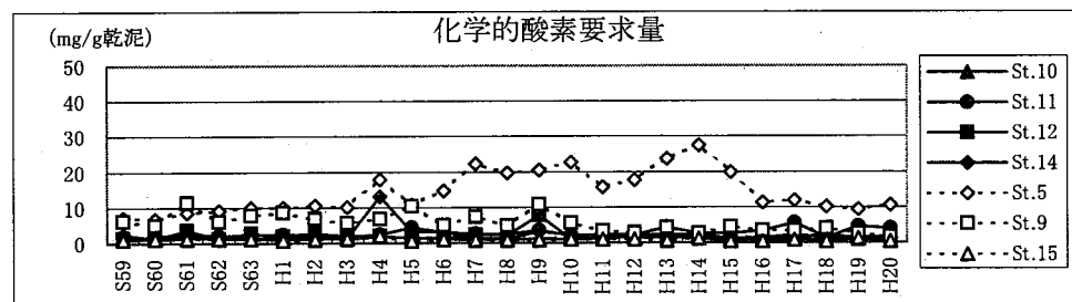
図III-2-2(2) 底質の評価点別経年変化
