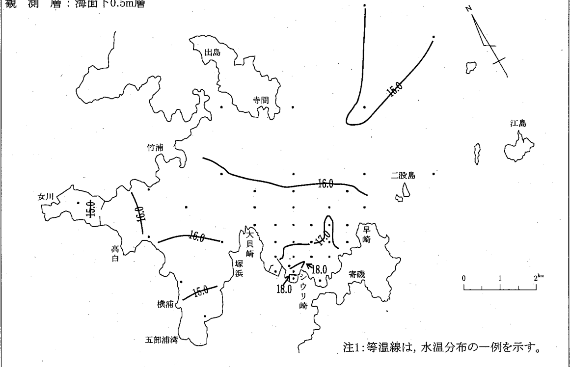
図-4-(2) 等温線
