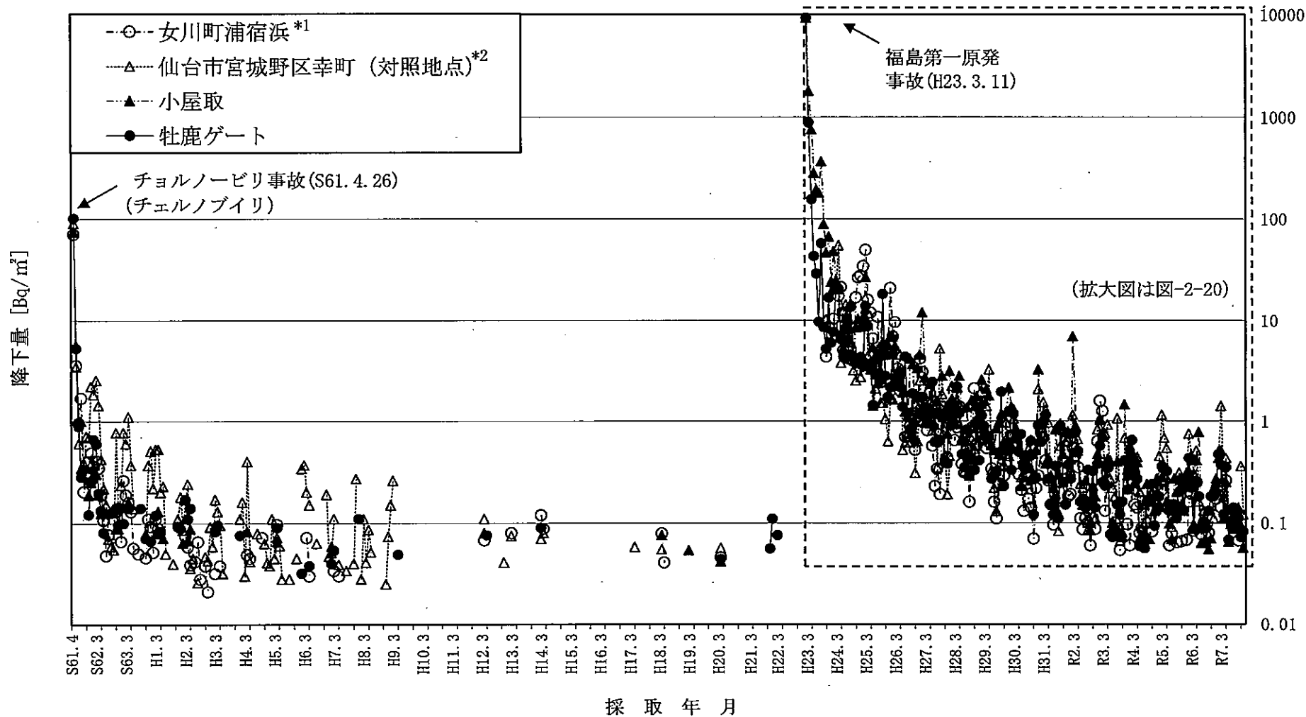
図-2-18 Cs-137の月間降下量の推移
