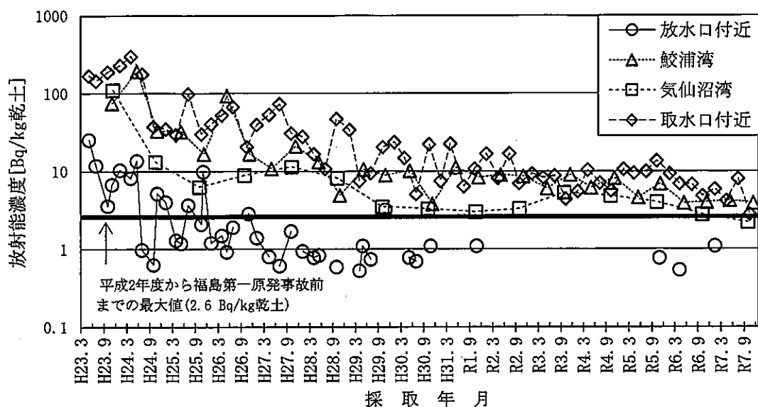
図-2-3-1 海底土のCs-137濃度の推移
