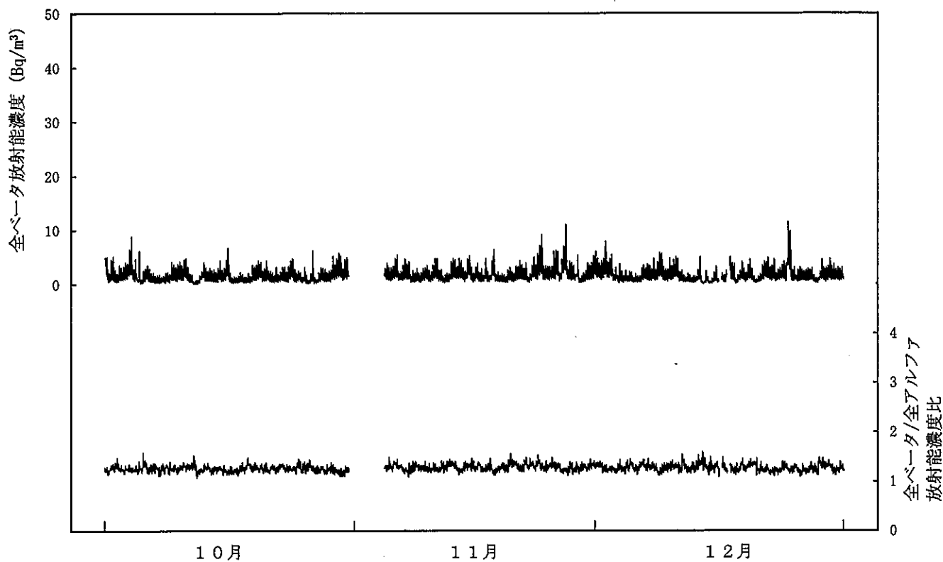
図－２－１６ 大気中の放射性物質の全ベータ放射能濃度及び 全ベータ／全アルファ放射能濃度比（飯子浜局）
