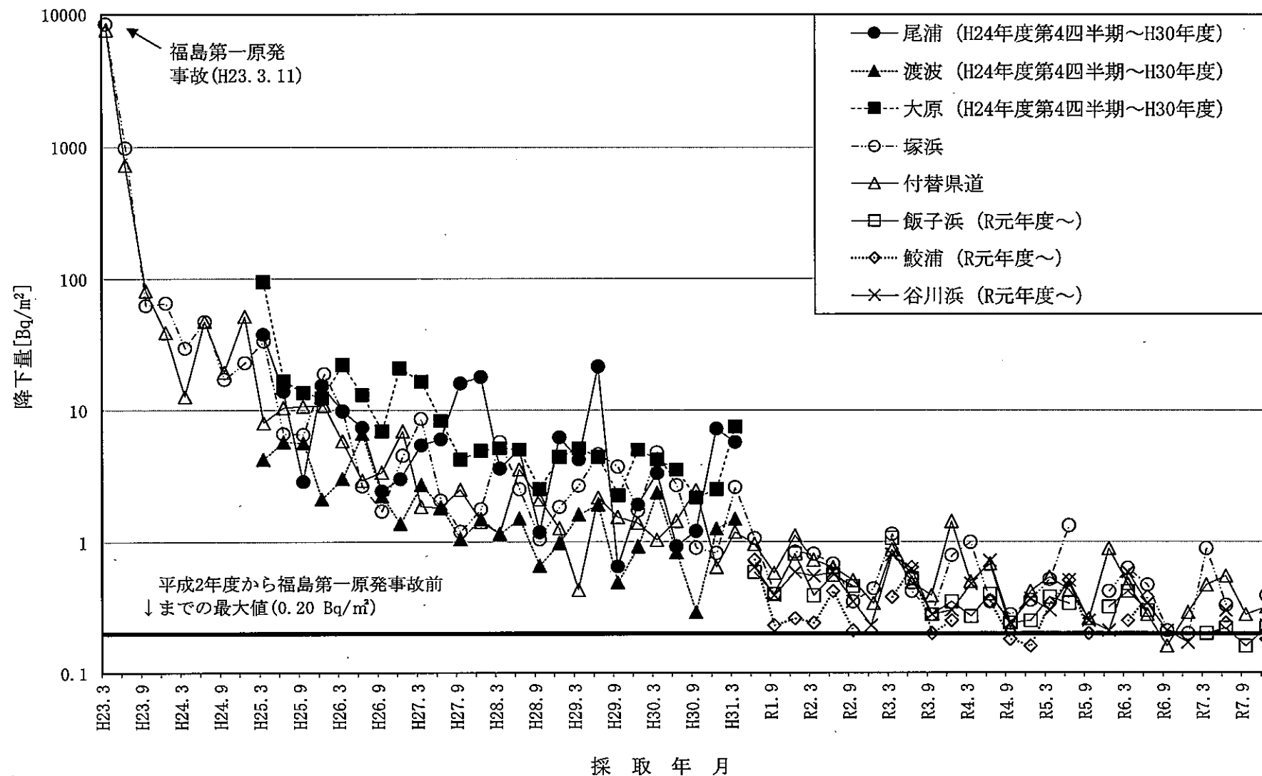
図－2－19 Cs-137の四半期間降下量の推移
