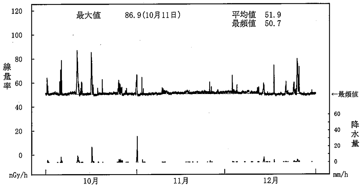
図－２－５ NaI(Tl)検出器による空間ガンマ線量率監視結果（鯨浦局）
